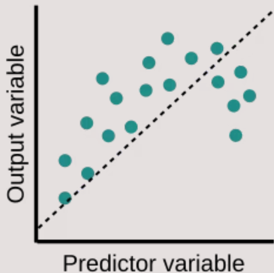
Subaprendizaje (underfitting)
