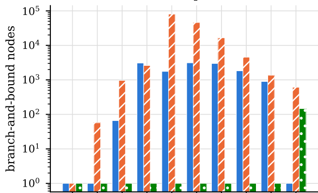
Makespan
