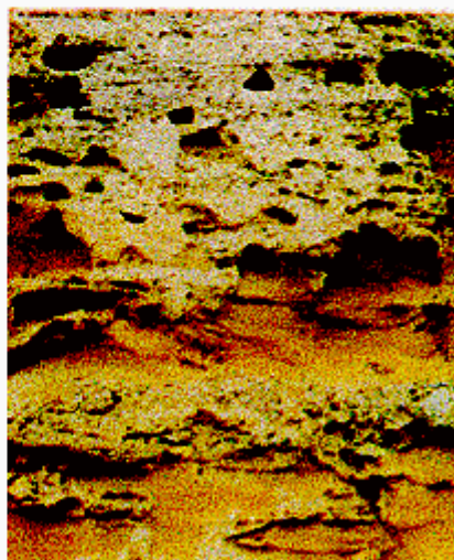
DETALLES DE LA SECUENCIA ESTRATIGRAFICA CARACTERISTICA DE LA FORMACION EL MILAGRO. CARRETERA A SAN FRANCISCO.
