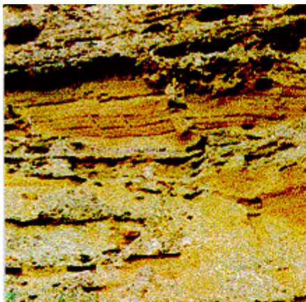
CERROS DE COTORRERA, EN LA FOTOCOMPOSICION ARRIBA (DIRECCION: ESTE) Y DETALLE DE LA ESTRATIGRAFIA ABAJO. POR ALLI ANDARIAN LOS PRIMEROS HABITANTES DE LA REGION, Y LOS INDIOS. SOBRE COTORRERA SE FUNDO MARACAIBO -FUESE ALFINGER, PACHECO O MALDONADO- Y MORALES IMPOTENTE FUE TESTIGO DE LA DERROTA DE SU FLOTA.
