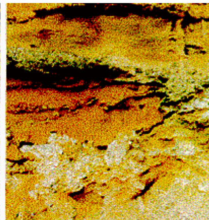
CERROS DE COTORRERA, EN LA FOTOCOMPOSICION ARRIBA (DIRECCION: ESTE) Y DETALLE DE LA ESTRATIGRAFIA ABAJO. POR ALLI ANDARIAN LOS PRIMEROS HABITANTES DE LA REGION, Y LOS INDIOS. SOBRE COTORRERA SE FUNDO MARACAIBO -FUESE ALFINGER, PACHECO O MALDONADO- Y MORALES IMPOTENTE FUE TESTIGO DE LA DERROTA DE SU FLOTA.
