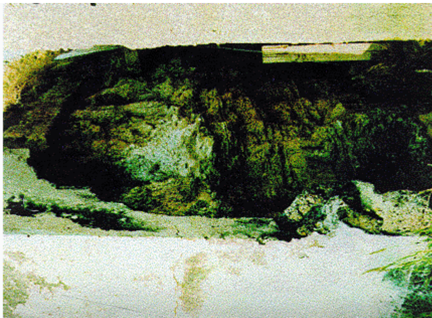
VENTANA PARA ENCONTRAR LA FORMACION EL MILAGRO, OCULTA EN ARAS DEL PROGRESO. A LA IZQUIERDA, EL MURO DONDE SE ASENTÓ UNA CASA, DEJANDO AL DESCUBIERTO CON RESPECTO LAS ARENISCAS FERRUGINOSAS DE EL MILAGRO, EN TODA SU EXTENSION; A LA DERECHA, EL MURO PROTECTOR DE UN MODERNO EDIFICIO, QUE TAPA POR COMPLETO LOS HORIZONTES DEL BANCO DE PIEDRAS.
