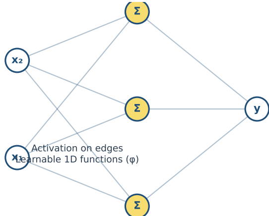
KAN
