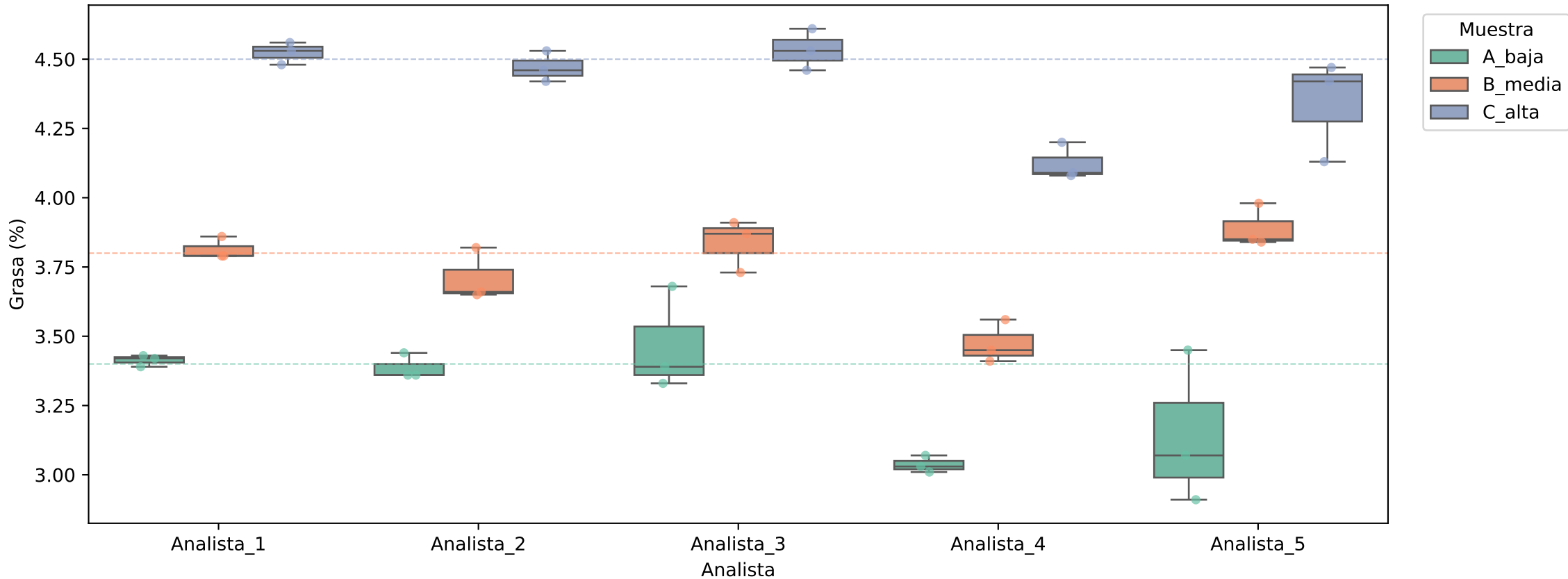
Resultados Gerber por analista y muestra (líneas discontinuas = valor de referencia)
