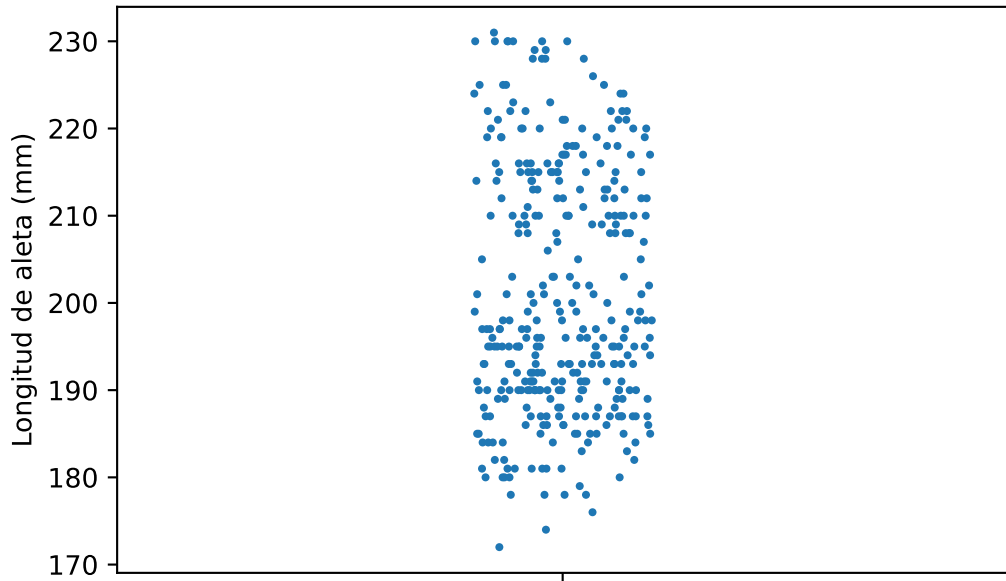
Dotplot con jitter: longitud de aleta
