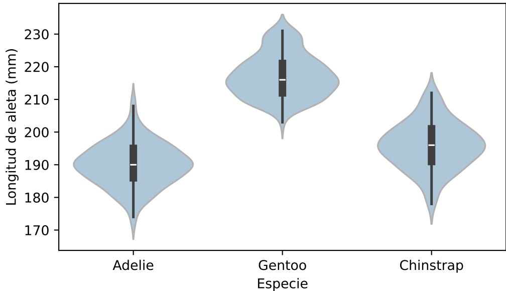
Violin plot por especie: longitud de aleta
