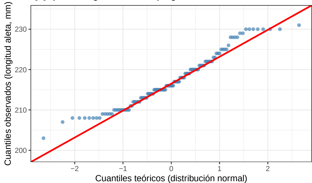
QQ-plot: Longitud aleta — pingüinos Gentoo
