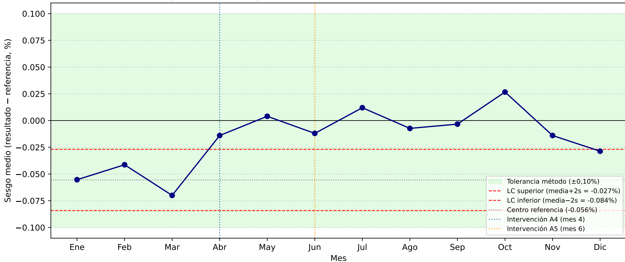
Seguimiento del sesgo del laboratorio — Método Gerber (muestra B, 3,8%)
