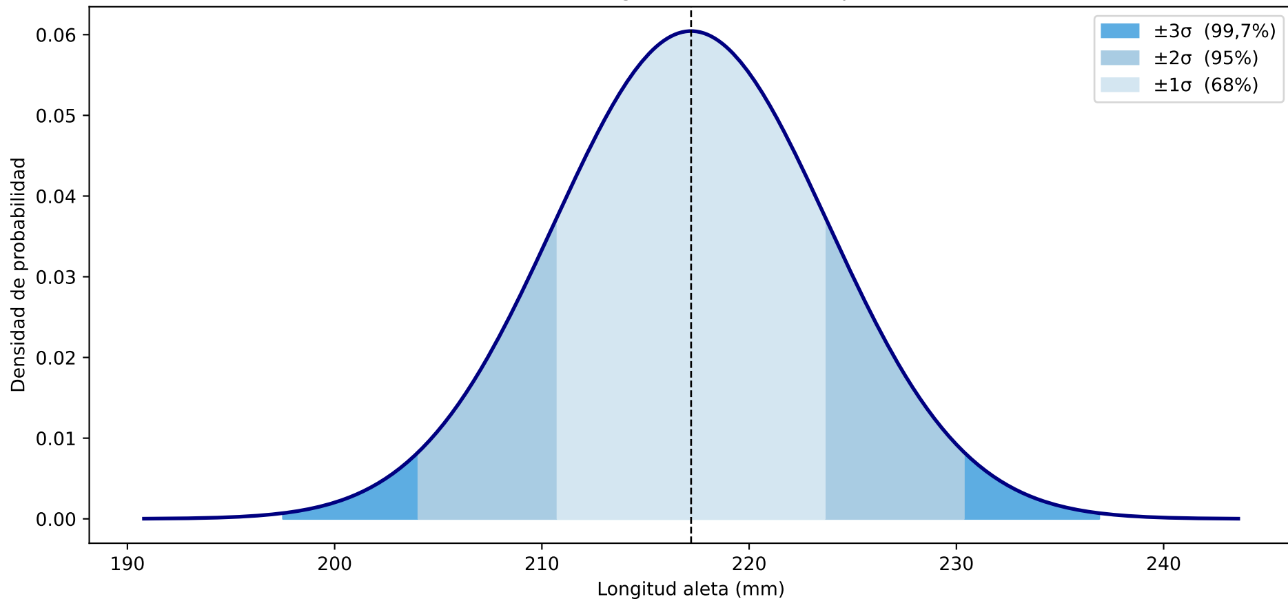
Distribución normal: longitud aleta Gentoo ( \mu=217.2 , \sigma=6.6 )
