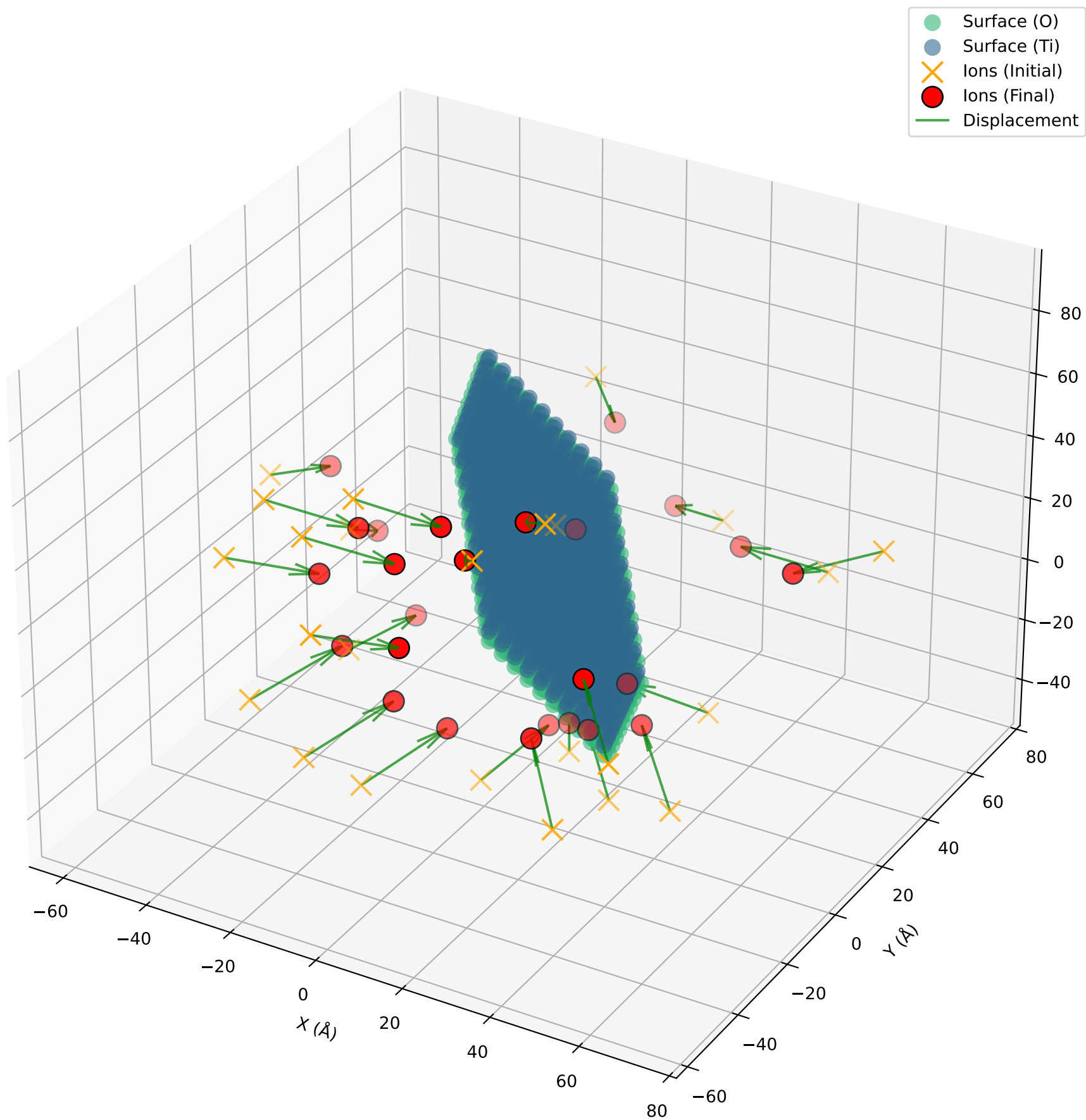
Initial and Final Ion Positions for TiO 2 _bulk_anatase_random_batch
