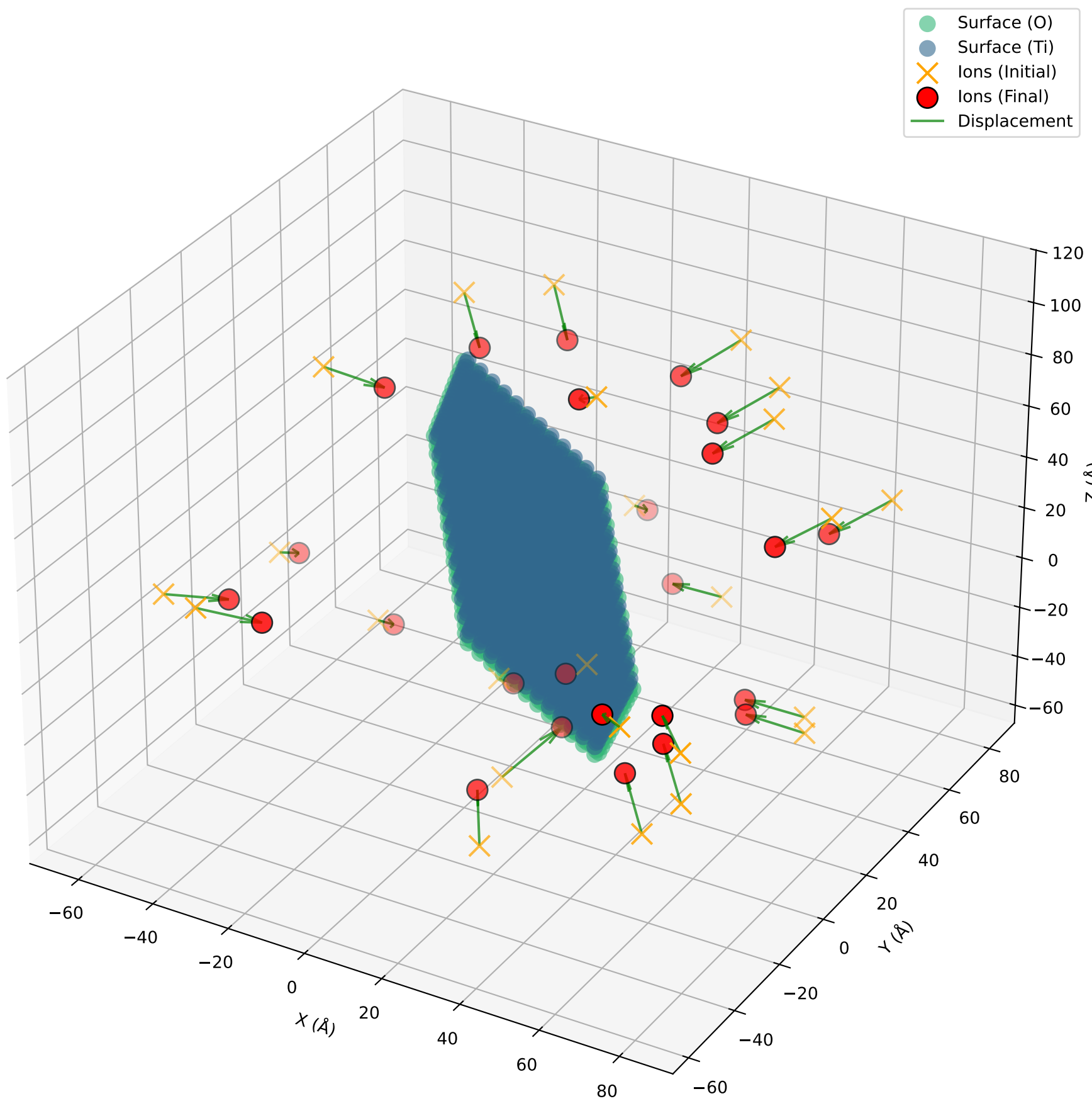
Initial and Final Ion Positions for TiO2_bulk_anatase_No_batch
