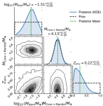
TOI-4438b
