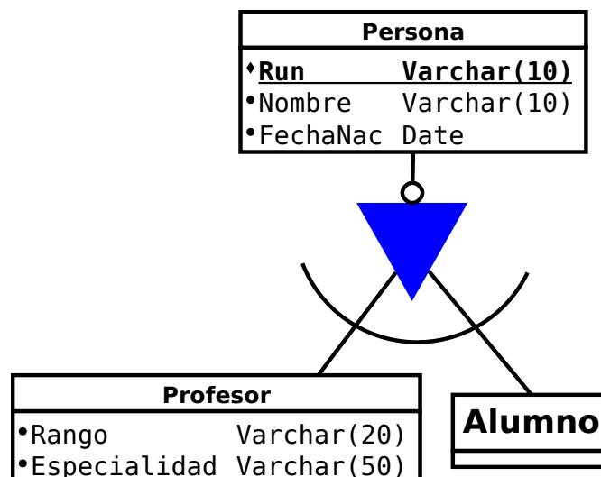
Figura 2.1: Herencia Persona
