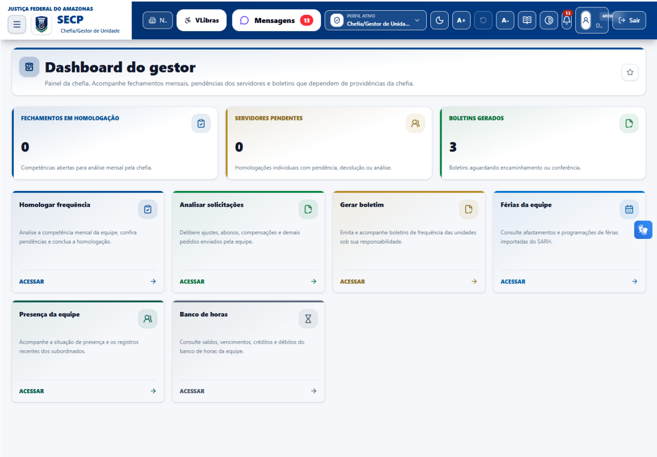
Figura 1 - Dashboard real do perfil Chefia/Gestor de Unidade no SECP.
