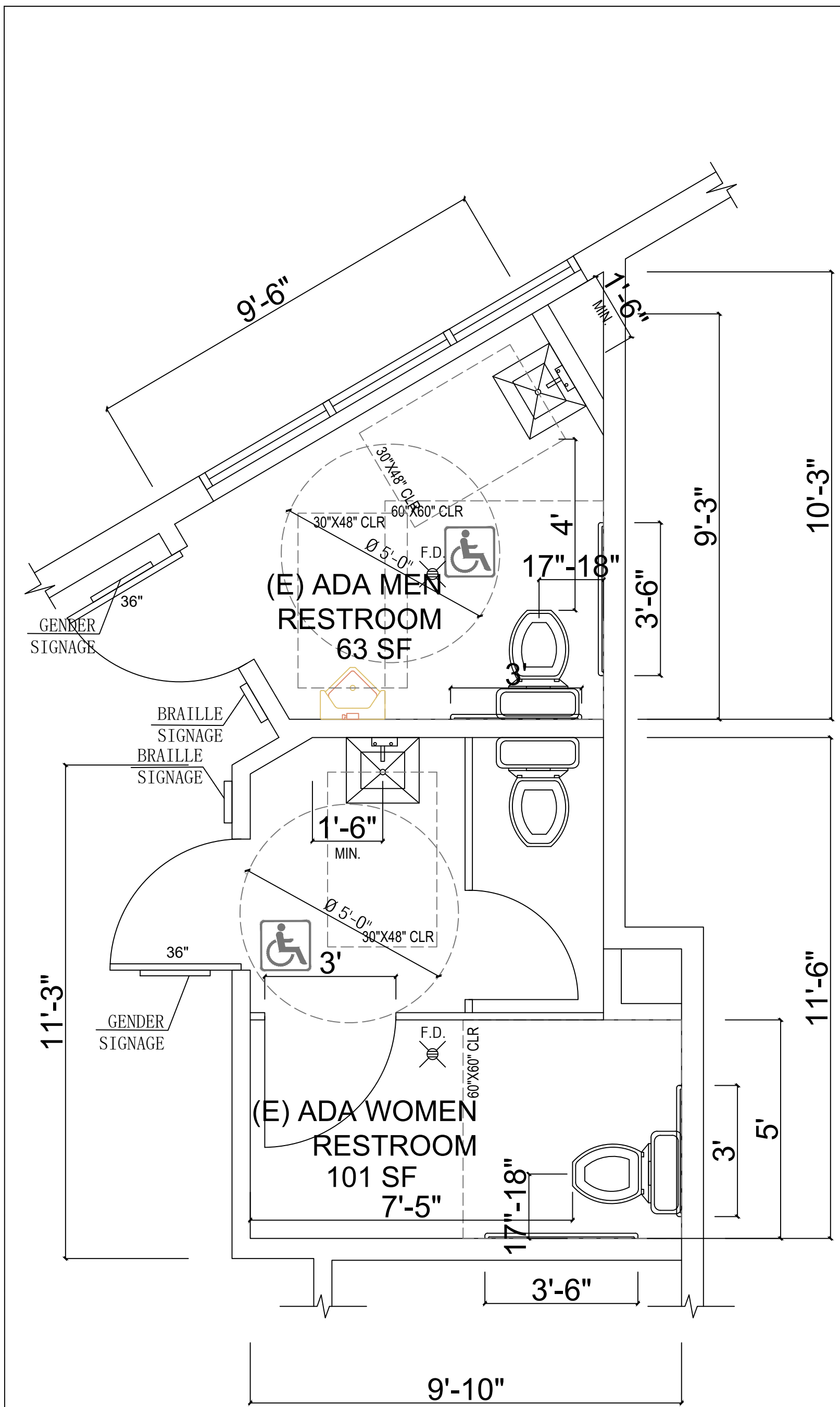
(E) RESTROOM PLAN VIEW SCALE N. T. S.
