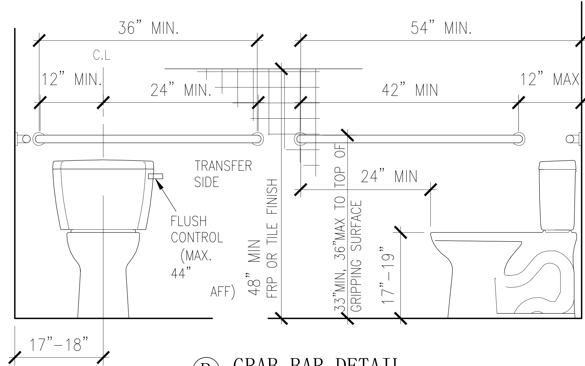
(B) GRAB BAR DETAIL SCALE N. T. S.
