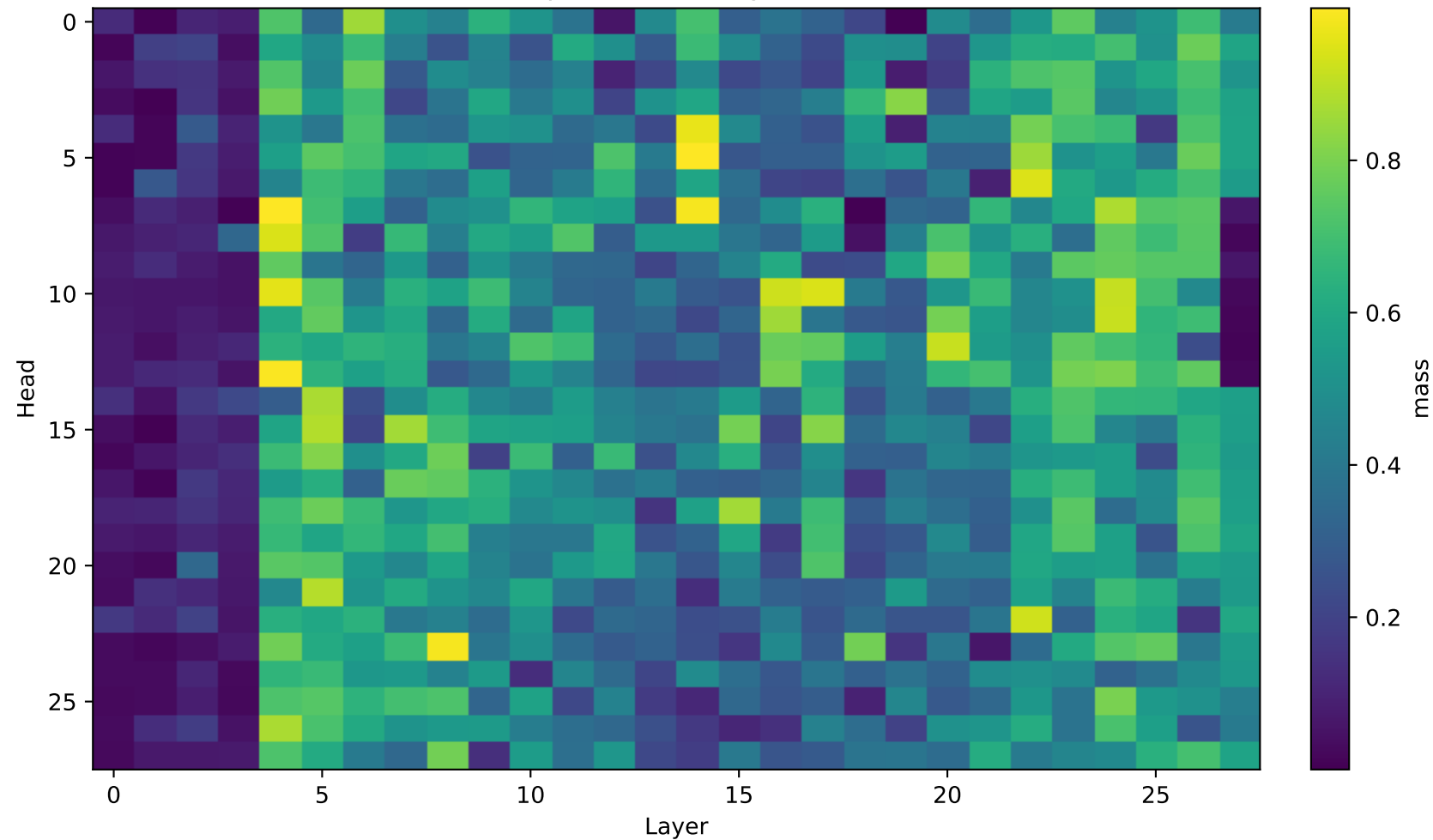
KVI: KV-prefix mass (layer \times head)
