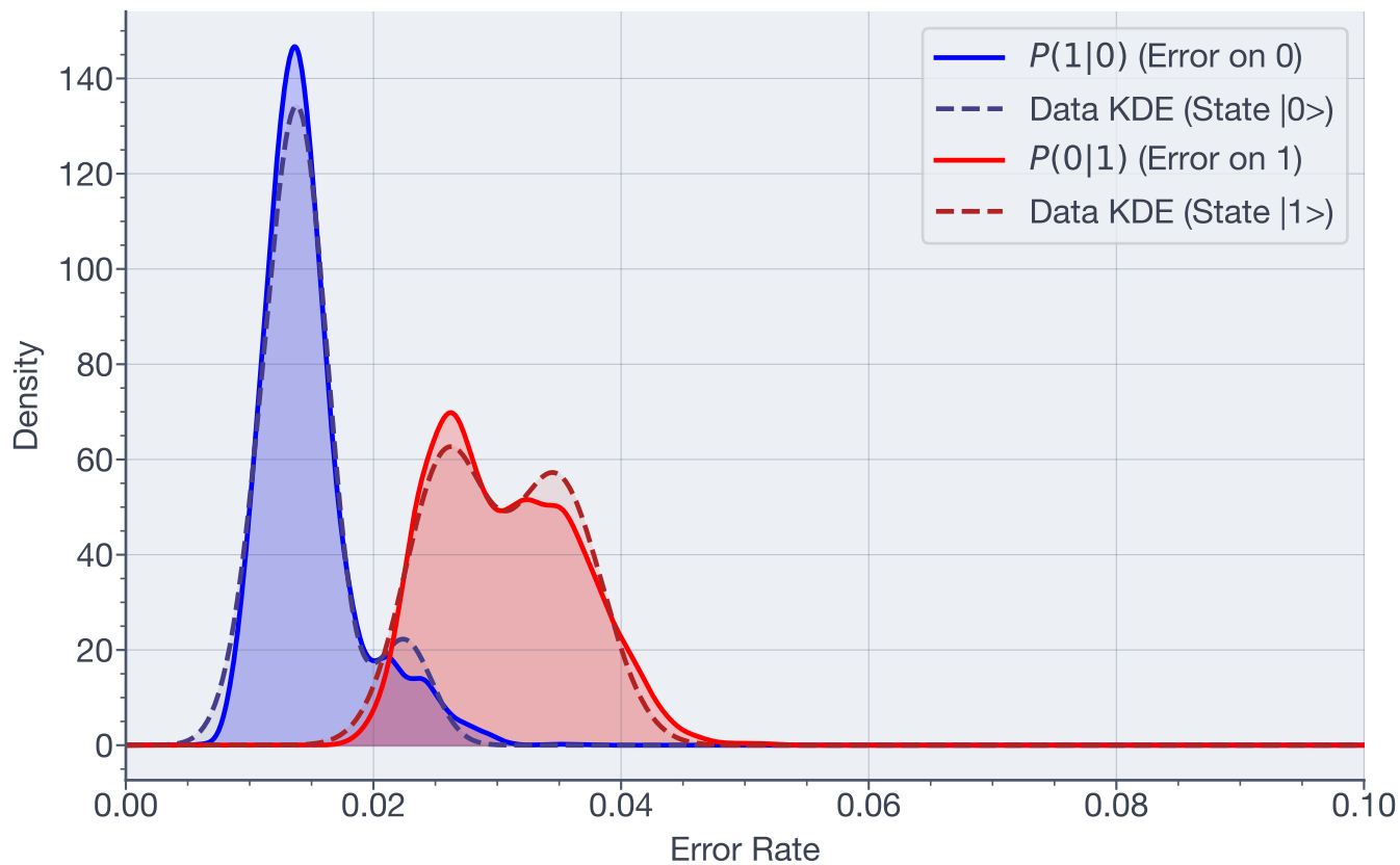
Posterior Error Distributions - Qubit 32
