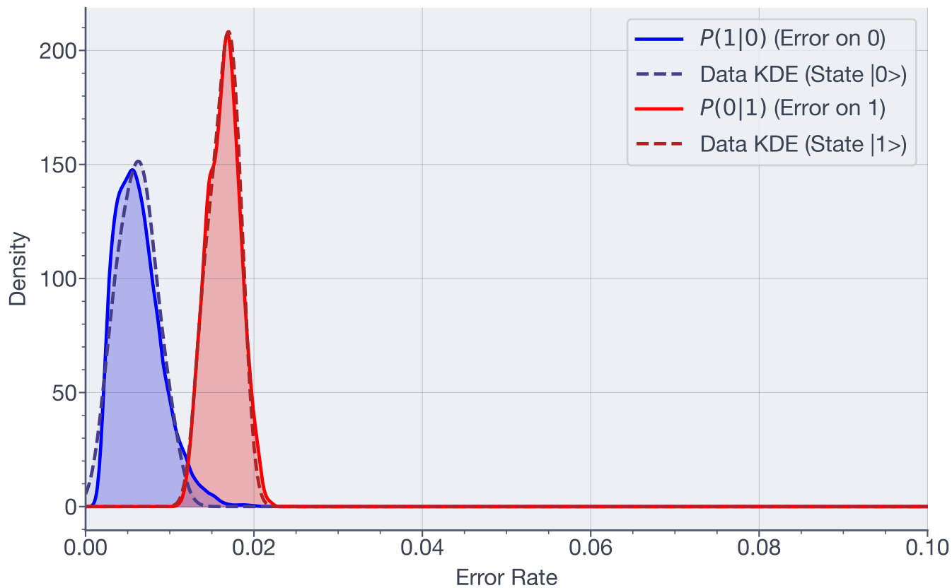
Posterior Error Distributions - Qubit 18
