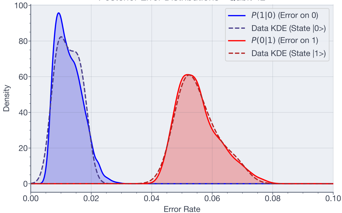
Posterior Error Distributions - Qubit 42
