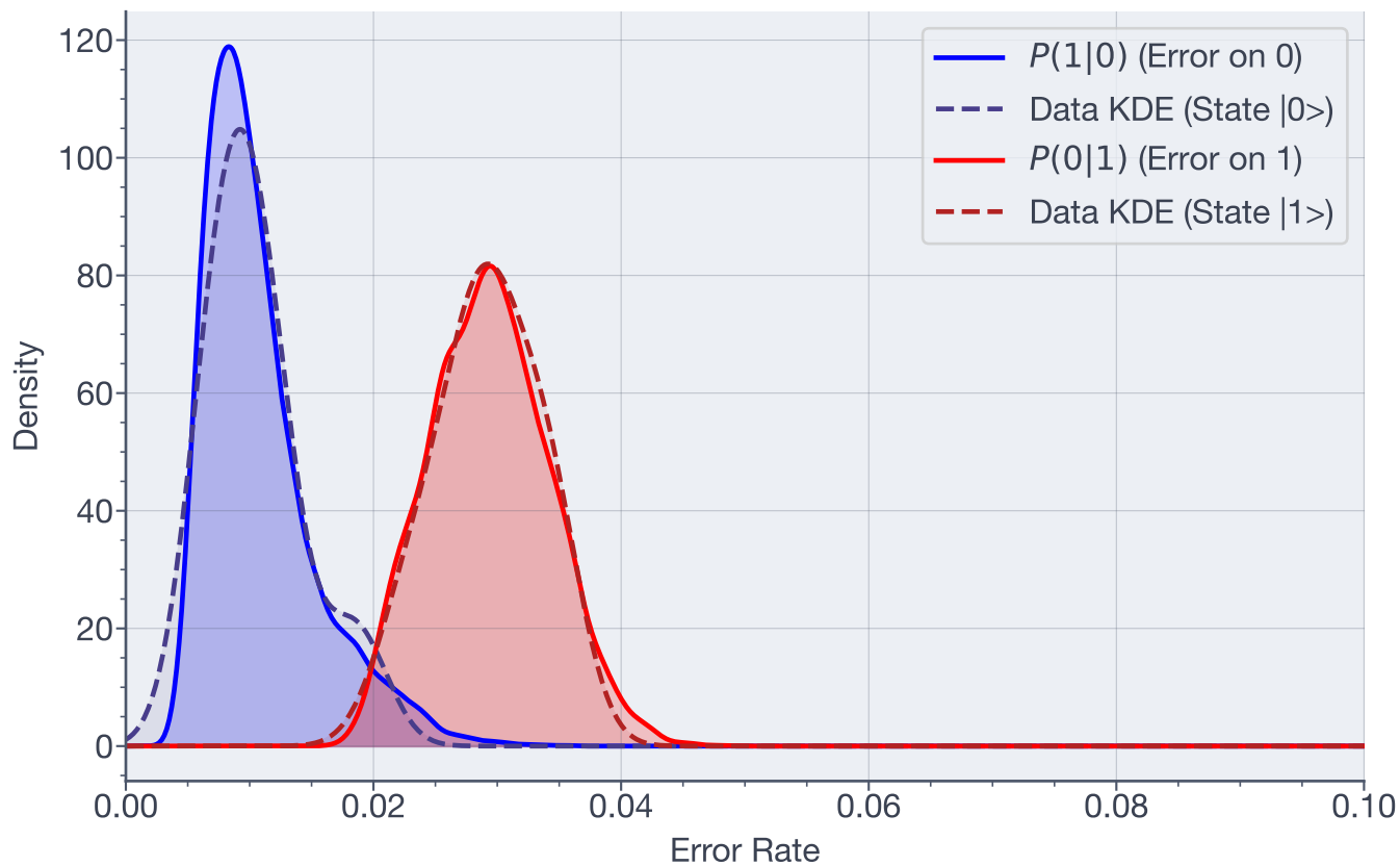
Posterior Error Distributions - Qubit 14
