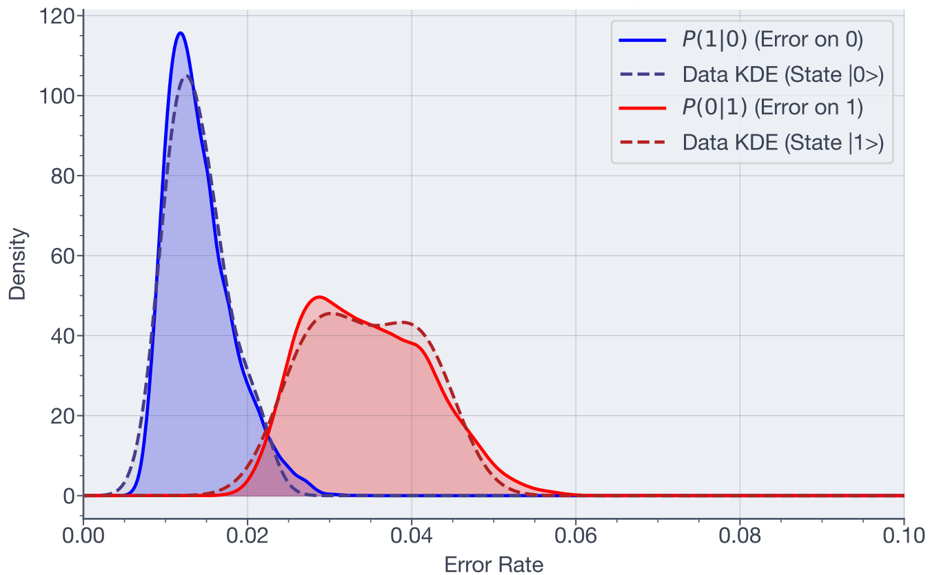
Posterior Error Distributions - Qubit 37
