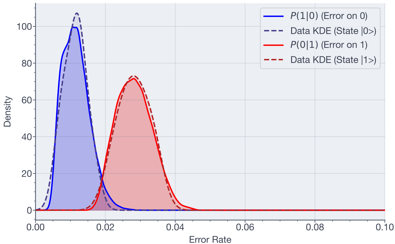
Posterior Error Distributions - Qubit 43
