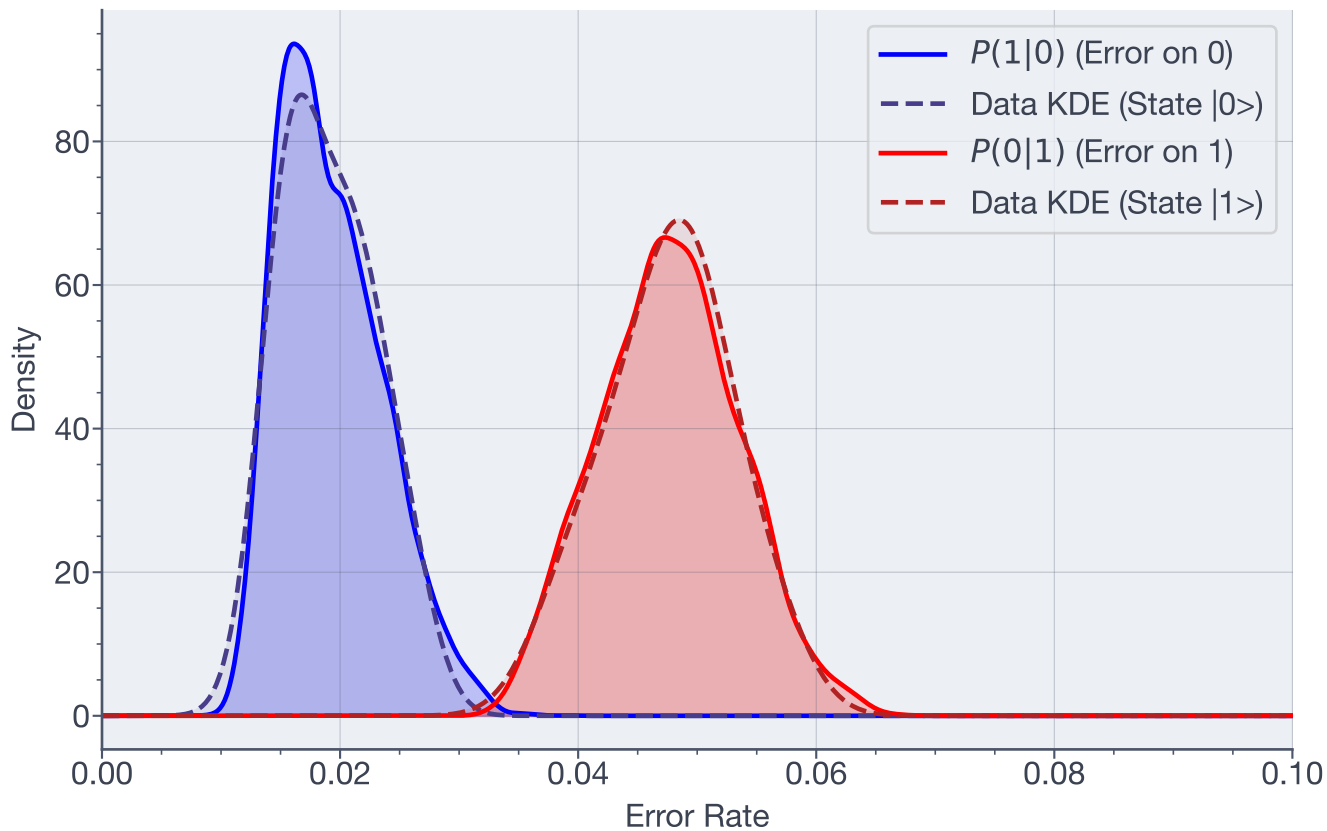
Posterior Error Distributions - Qubit 5
