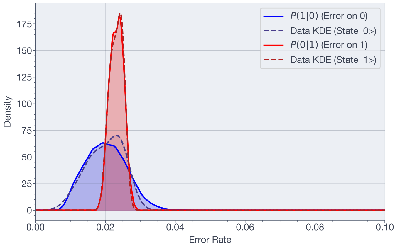
Posterior Error Distributions - Qubit 22
