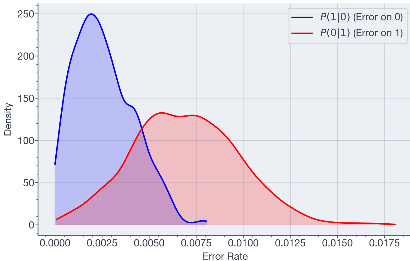
Posterior Error Distributions - Qubit 0
