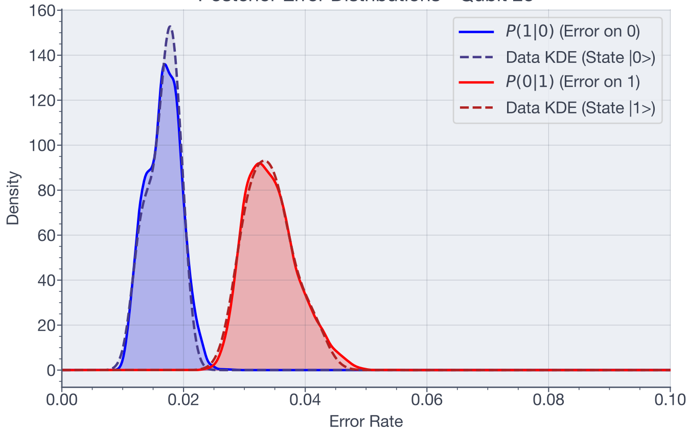
Posterior Error Distributions - Qubit 25
