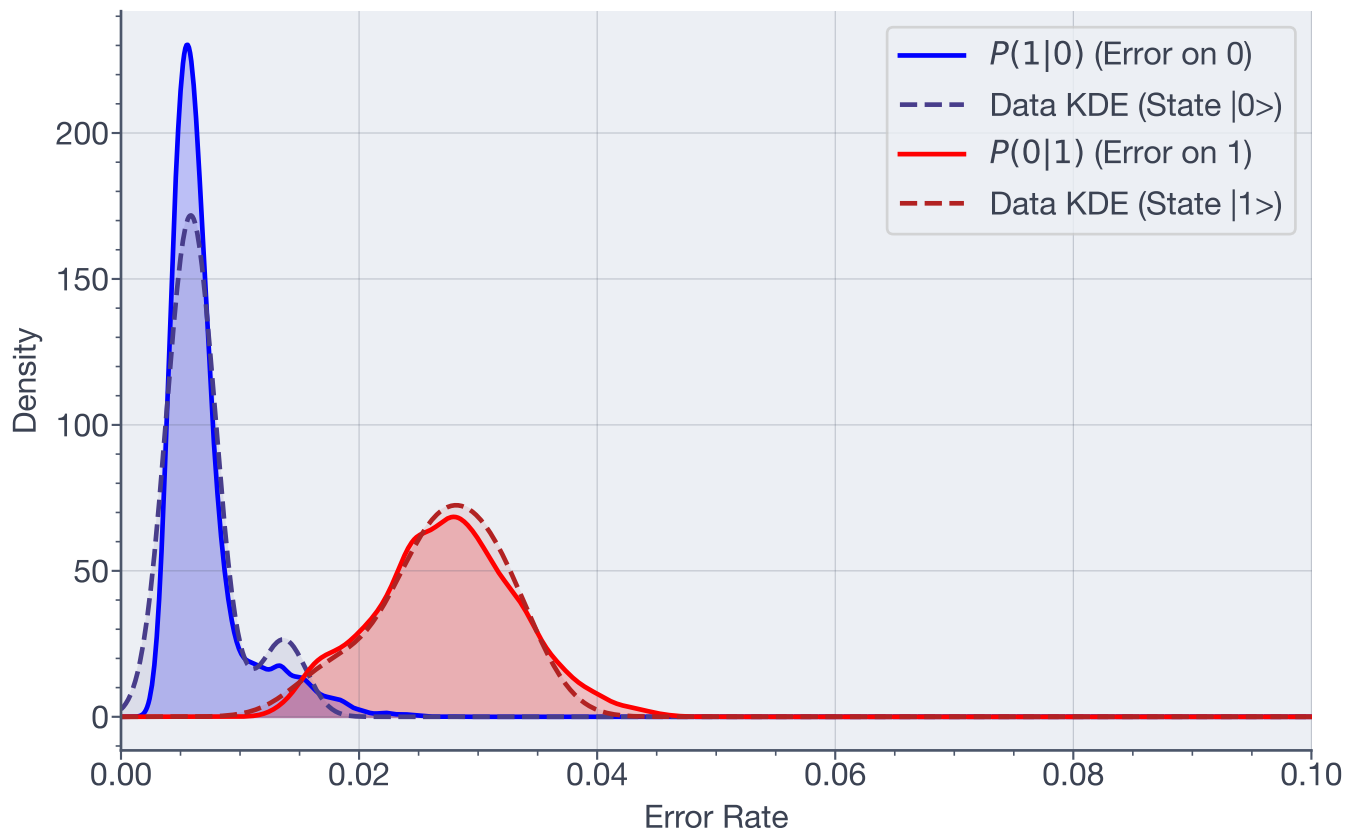
Posterior Error Distributions - Qubit 49
