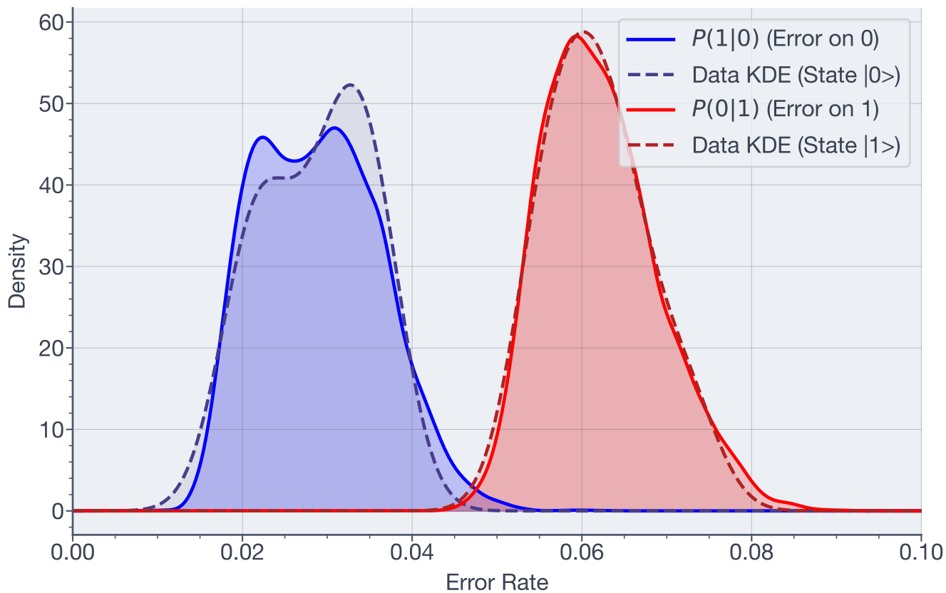
Posterior Error Distributions - Qubit 54
