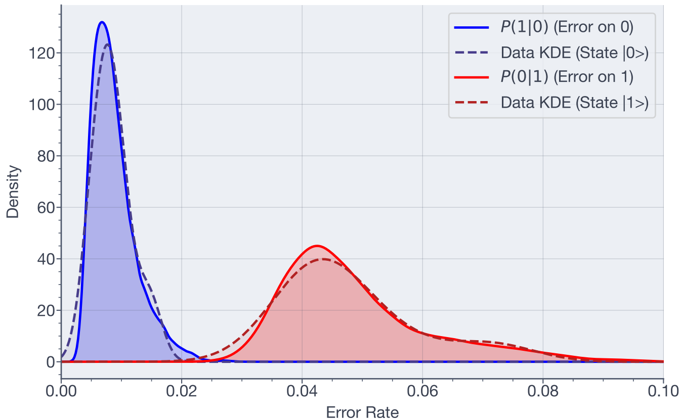
Posterior Error Distributions - Qubit 24
