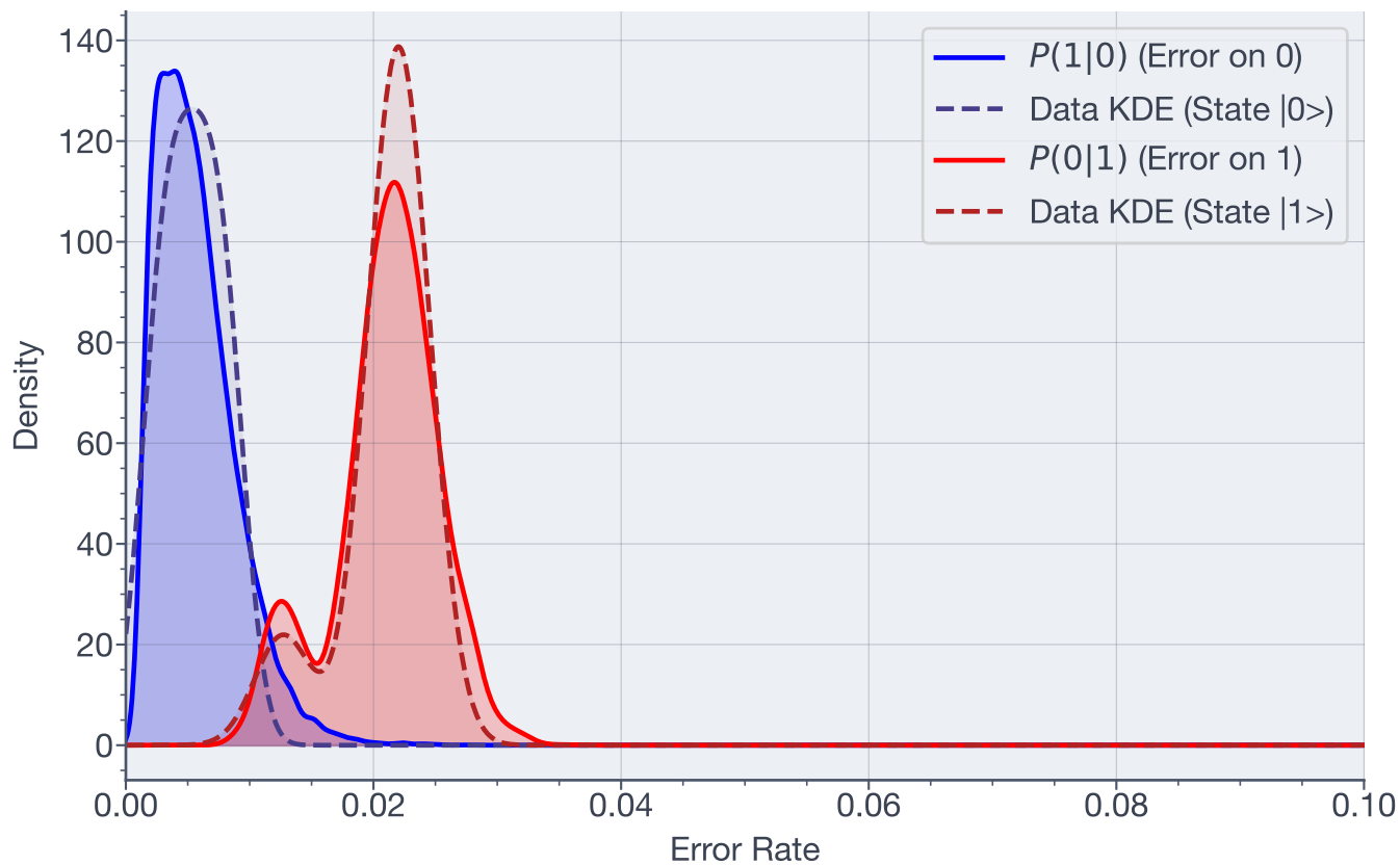
Posterior Error Distributions - Qubit 34
