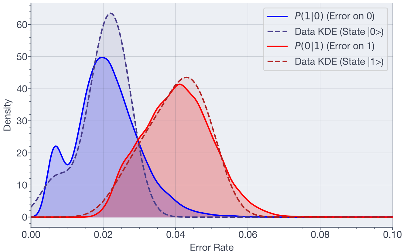
Posterior Error Distributions - Qubit 39
