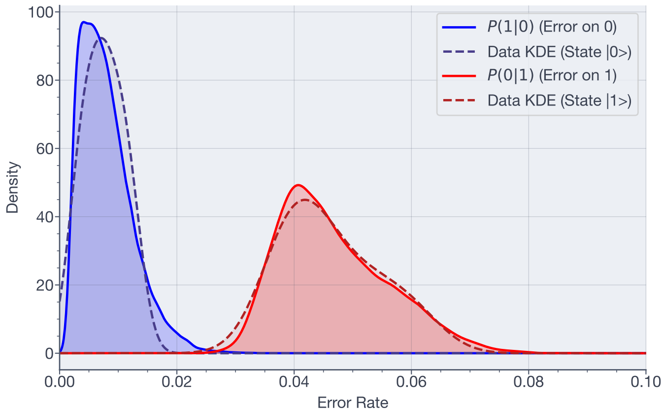
Posterior Error Distributions - Qubit 47
