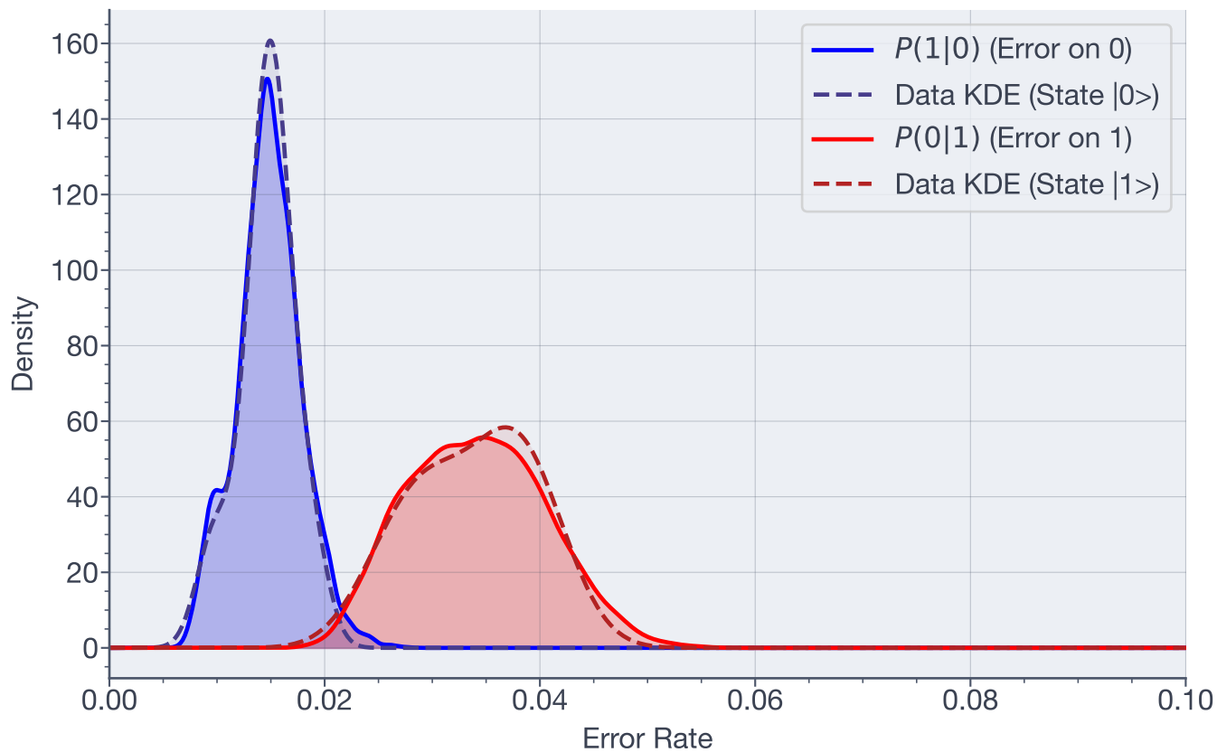
Posterior Error Distributions - Qubit 10
