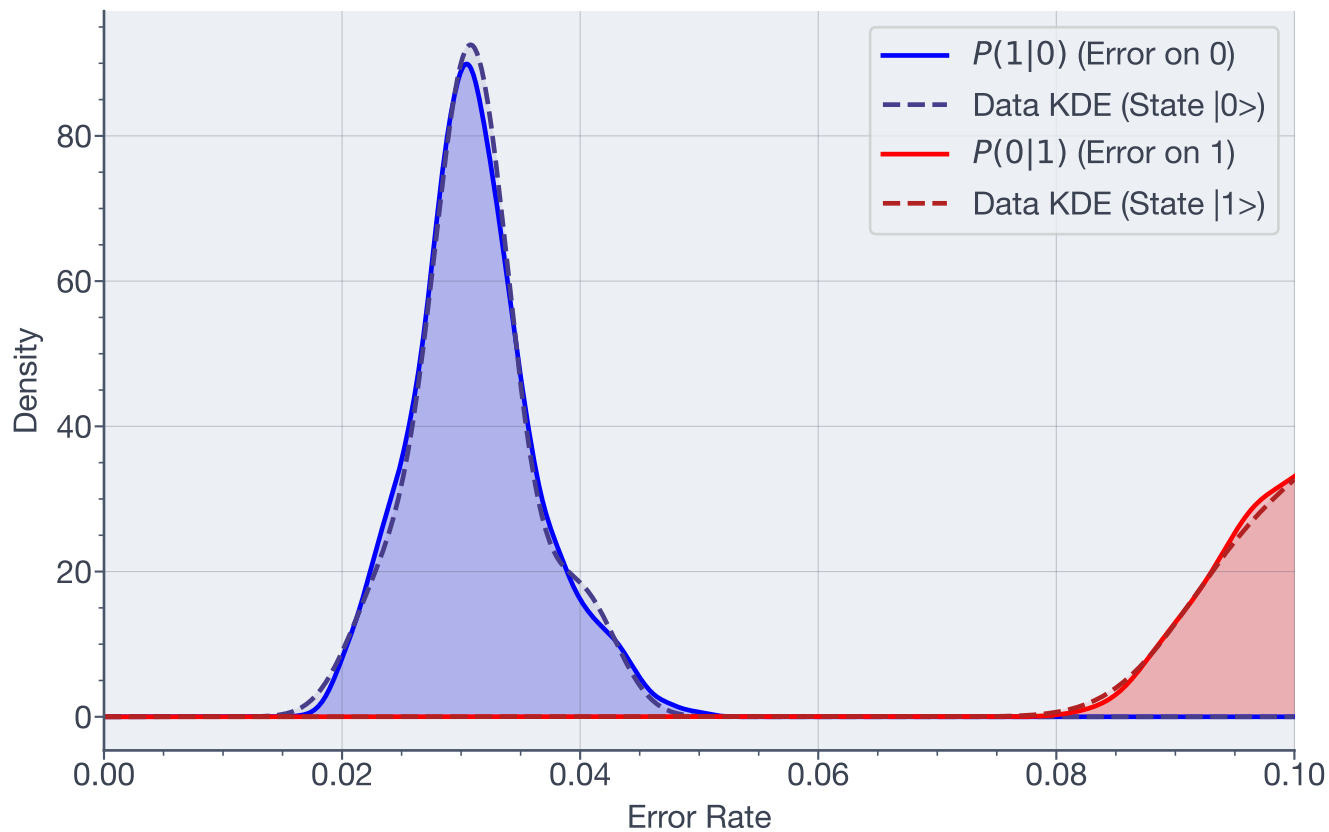
Posterior Error Distributions - Qubit 44
