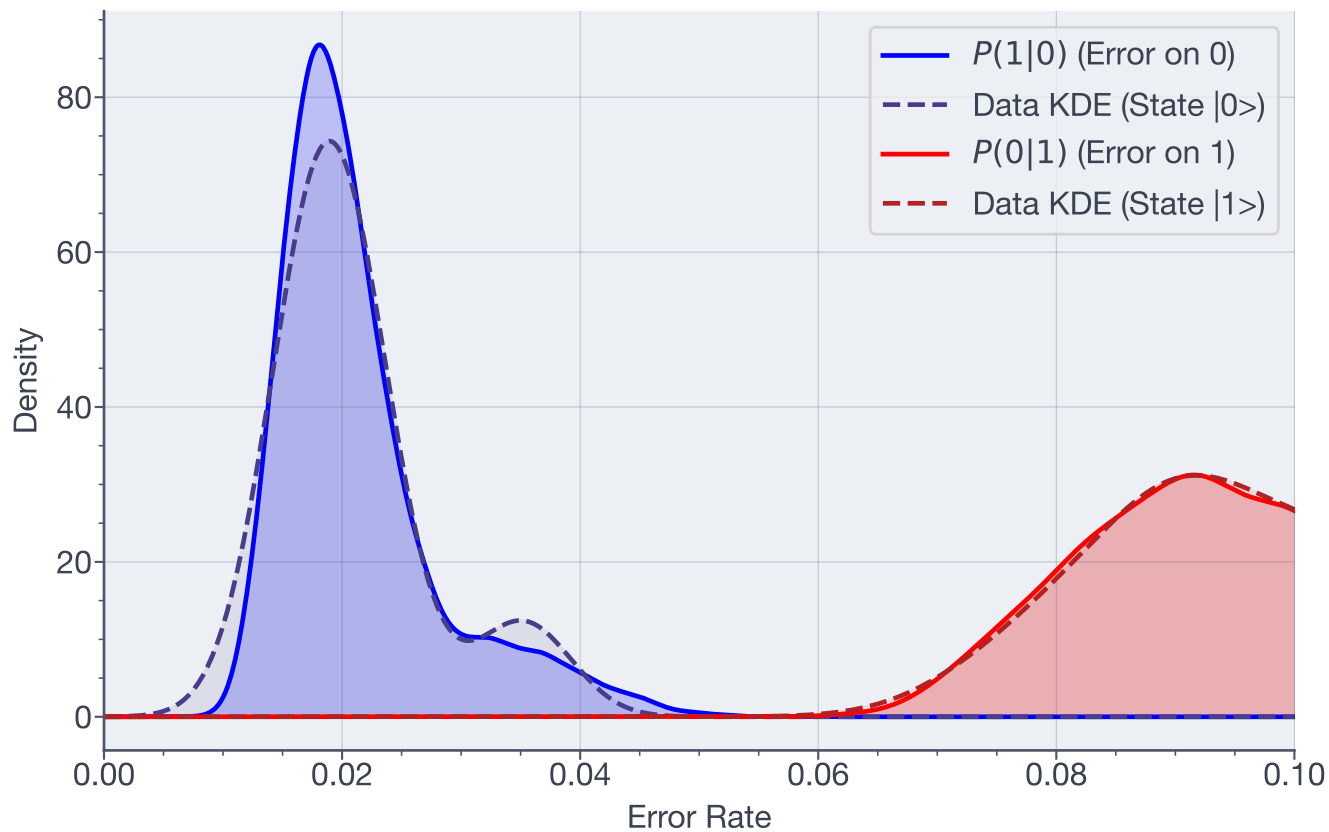
Posterior Error Distributions - Qubit 48
