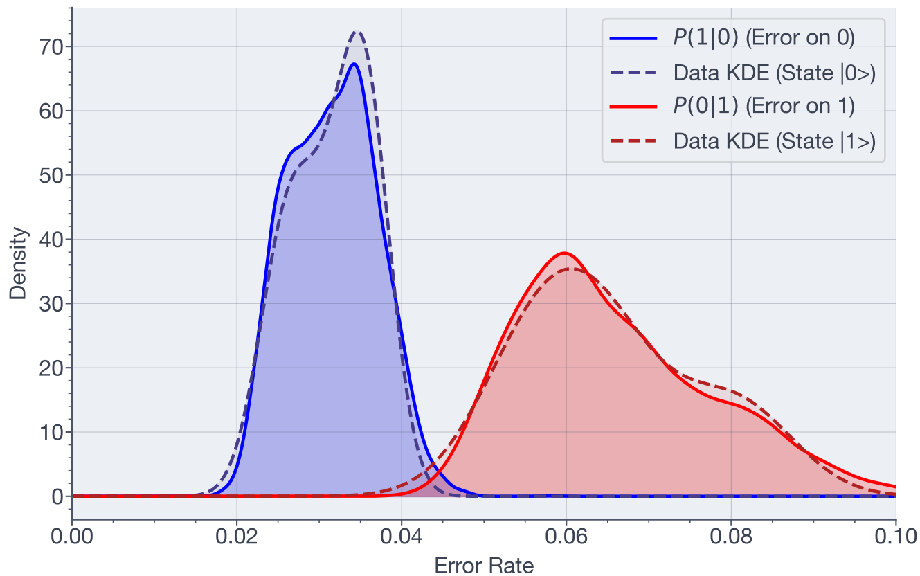
Posterior Error Distributions - Qubit 29
