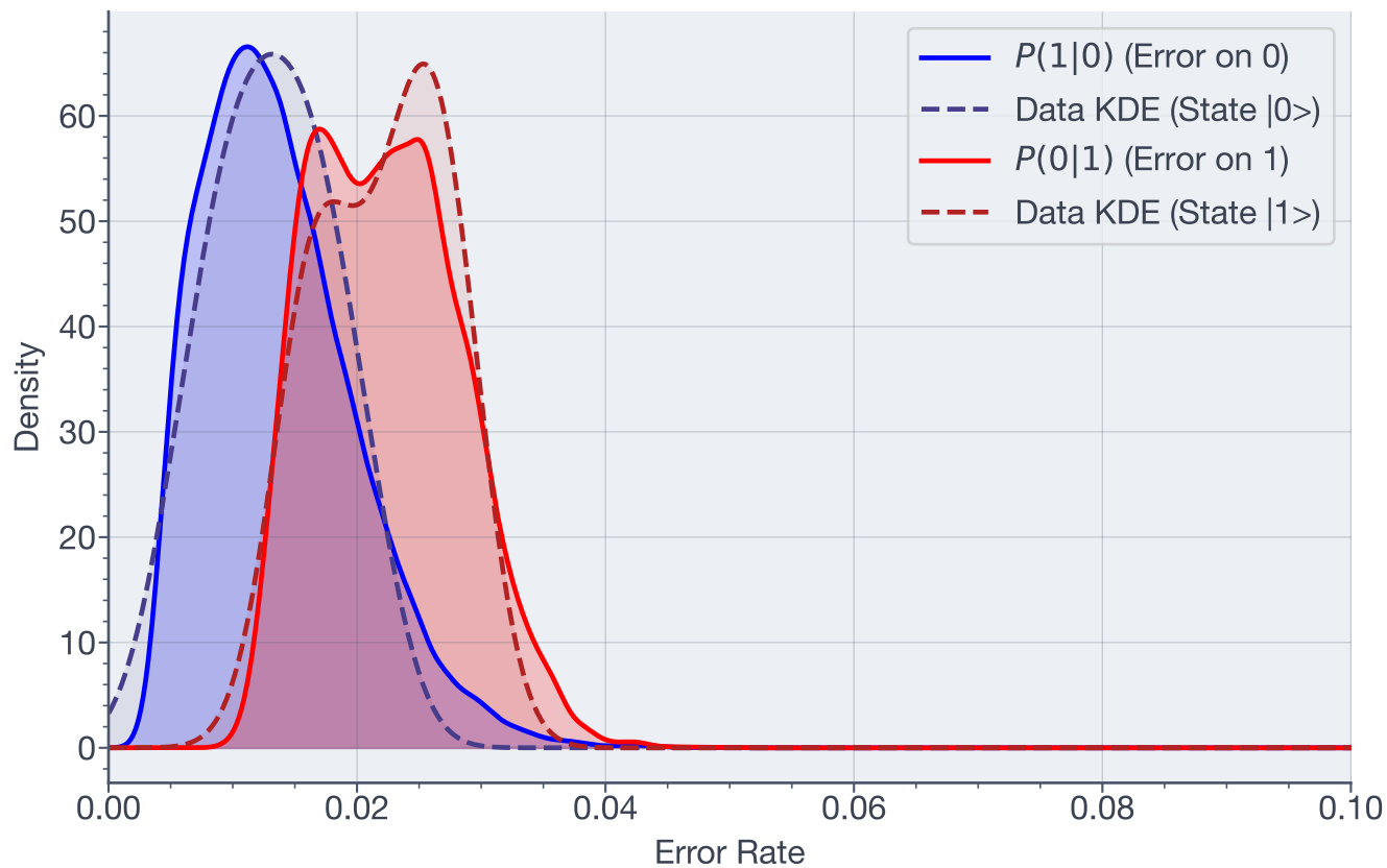
Posterior Error Distributions - Qubit 50
