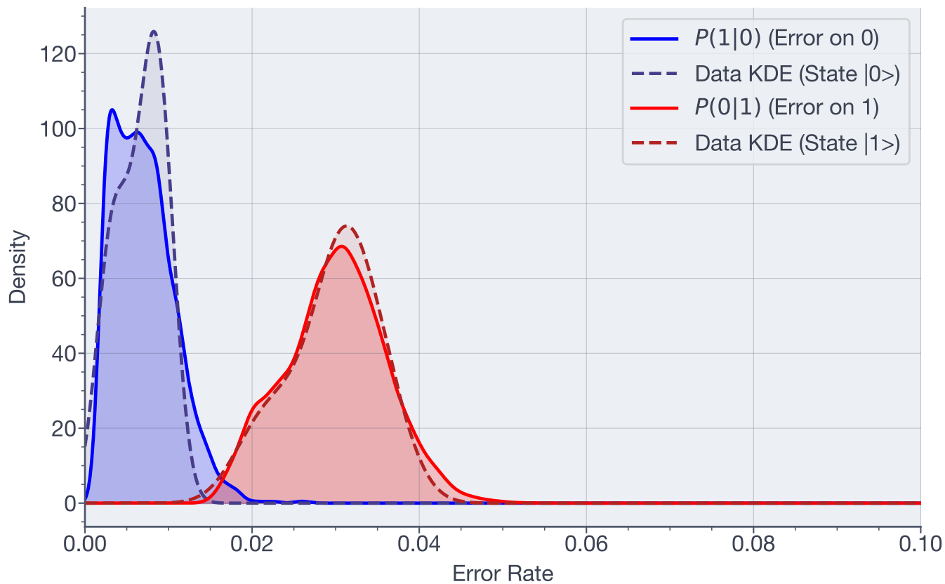
Posterior Error Distributions - Qubit 53
