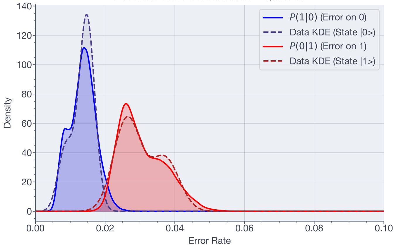
Posterior Error Distributions - Qubit 19
