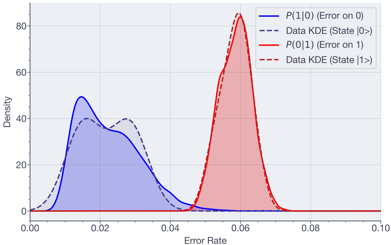
Posterior Error Distributions - Qubit 7
