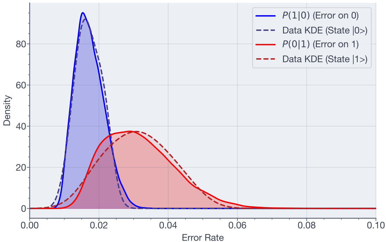
Posterior Error Distributions - Qubit 27
