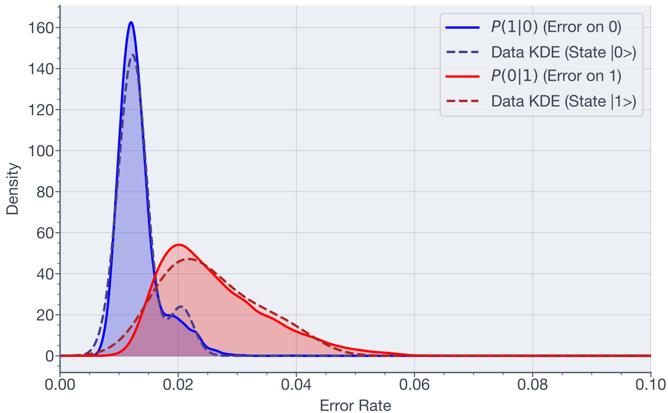
Posterior Error Distributions - Qubit 20
