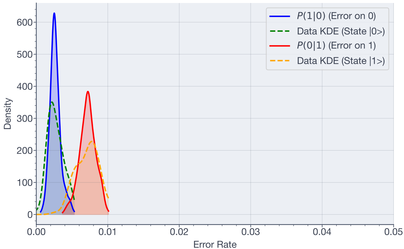
Posterior Error Distributions - Qubit 0
