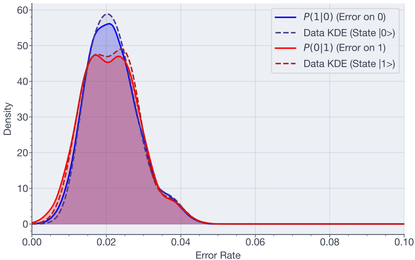
Posterior Error Distributions - Qubit 1
