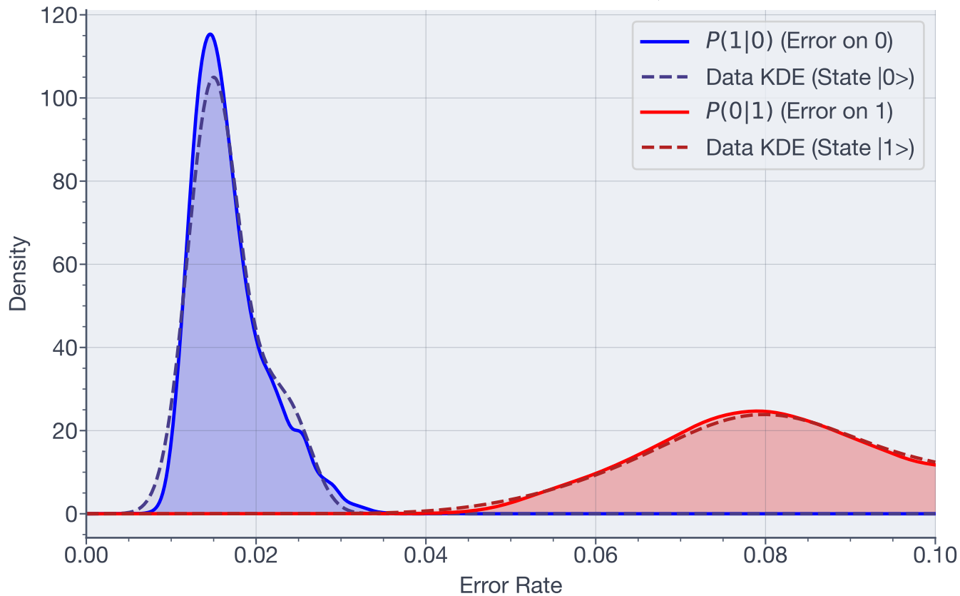
Posterior Error Distributions - Qubit 51
