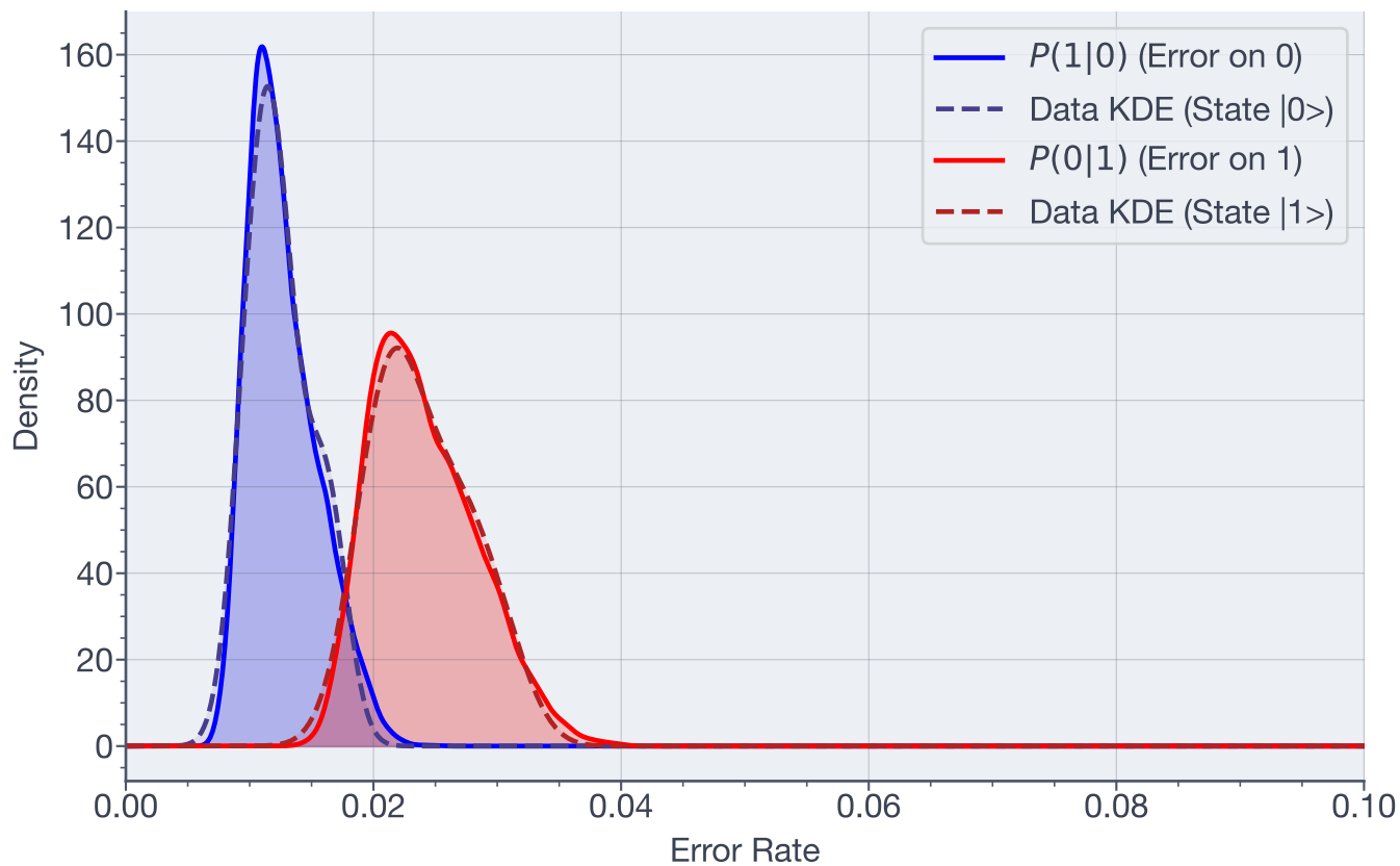
Posterior Error Distributions - Qubit 6
