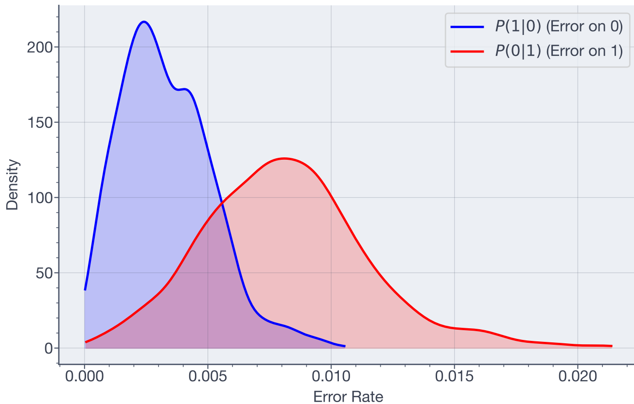
Posterior Error Distributions - Qubit 1
