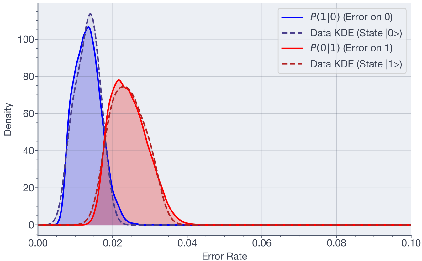
Posterior Error Distributions - Qubit 21
