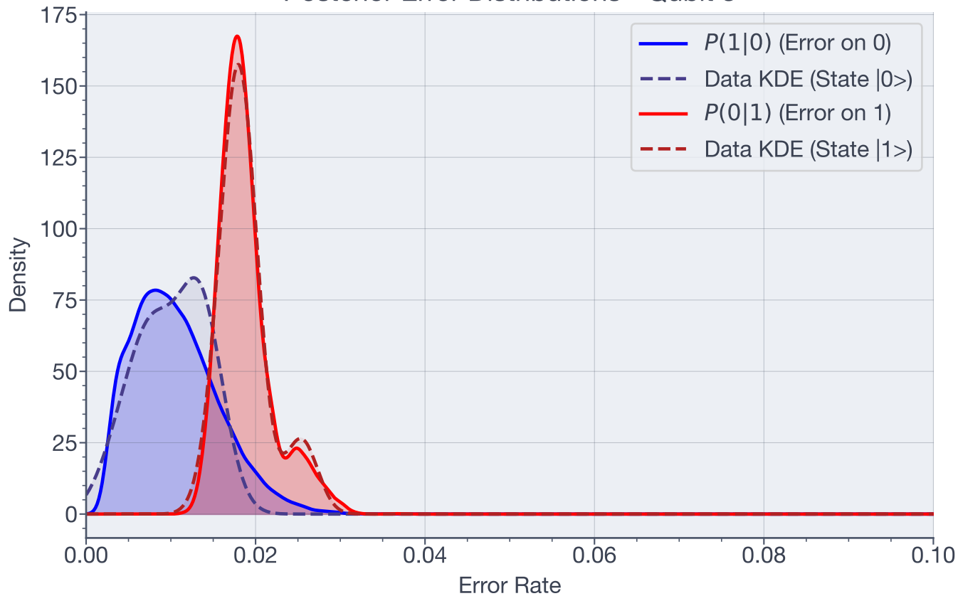
Posterior Error Distributions - Qubit 3
