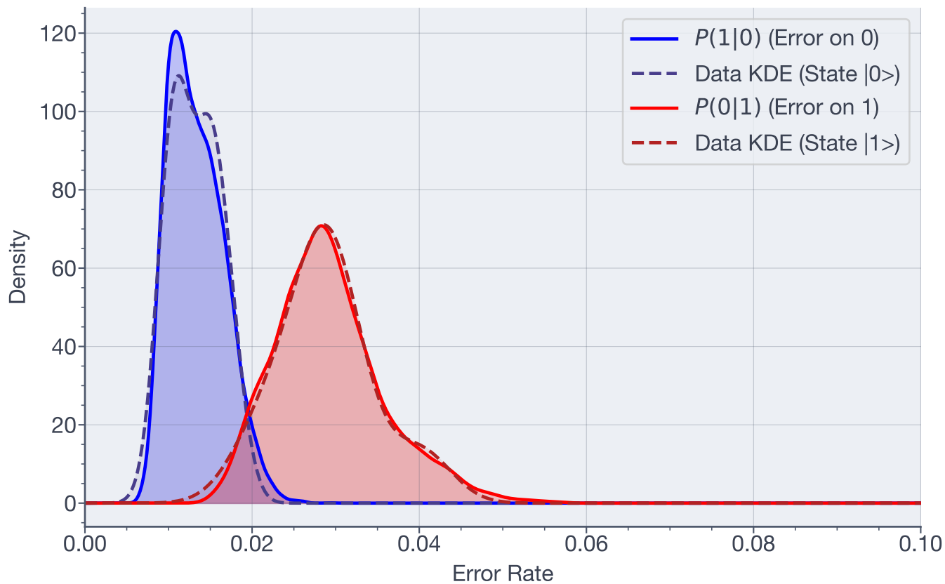
Posterior Error Distributions - Qubit 35
