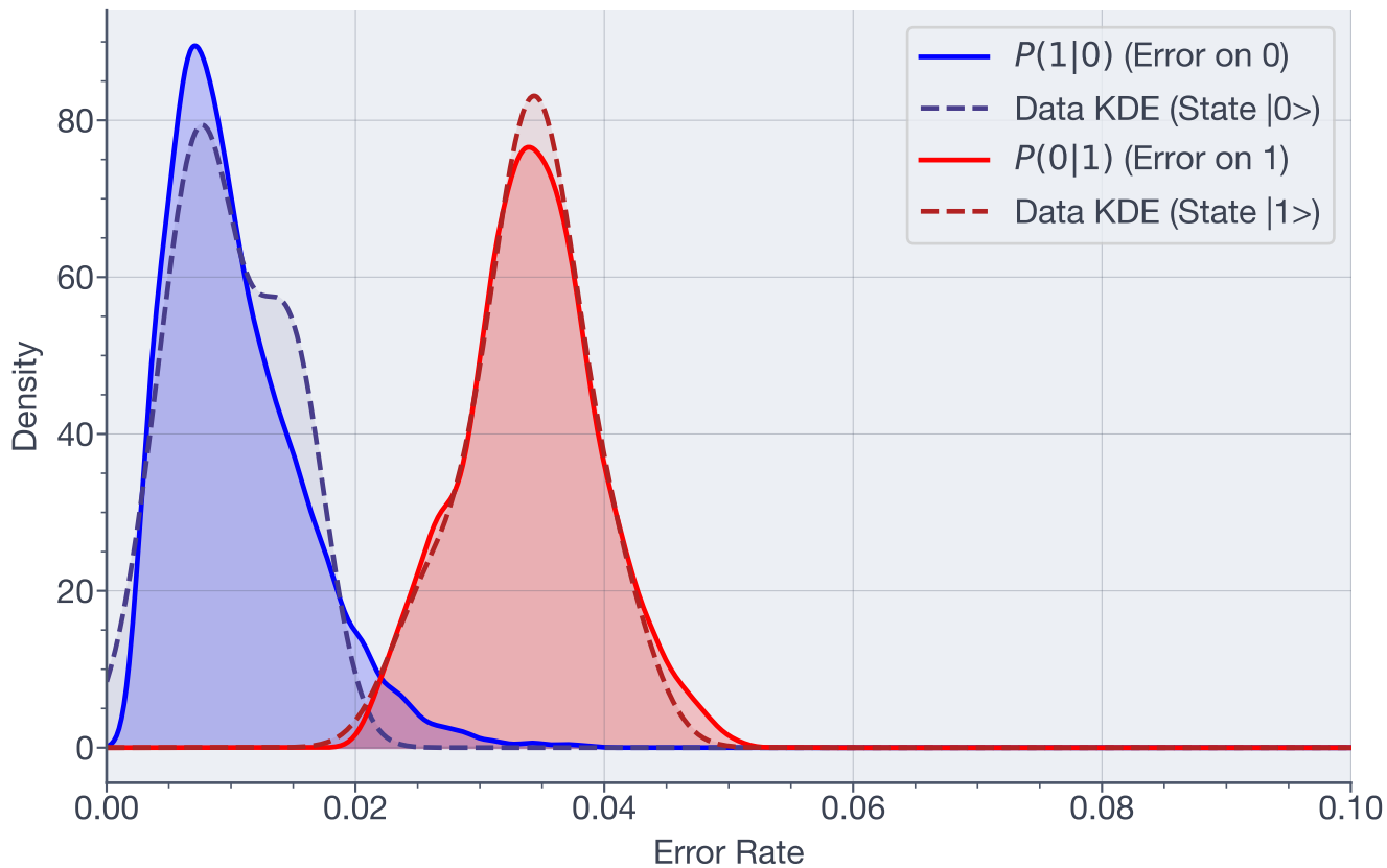
Posterior Error Distributions - Qubit 15
