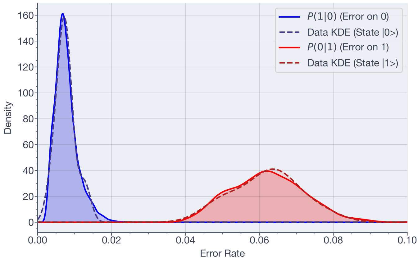
Posterior Error Distributions - Qubit 52
