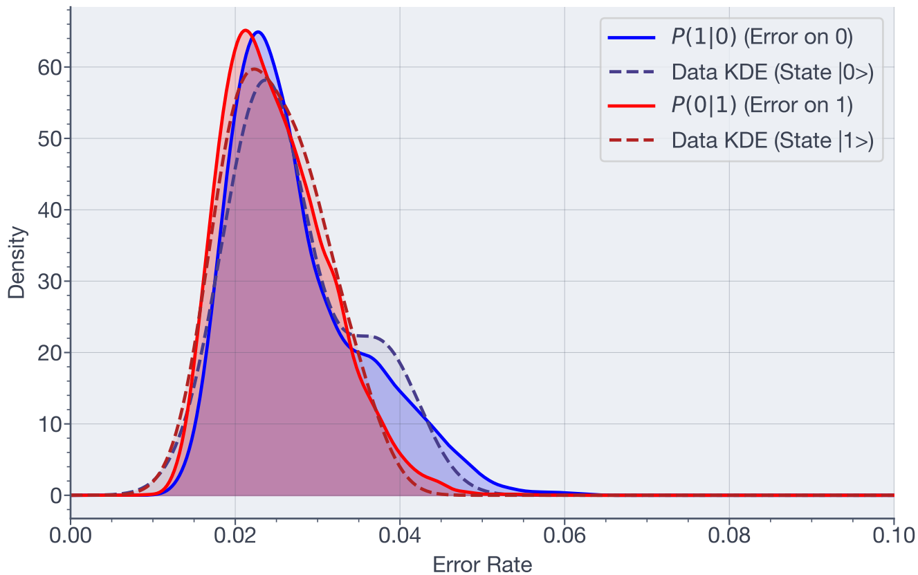
Posterior Error Distributions - Qubit 45
