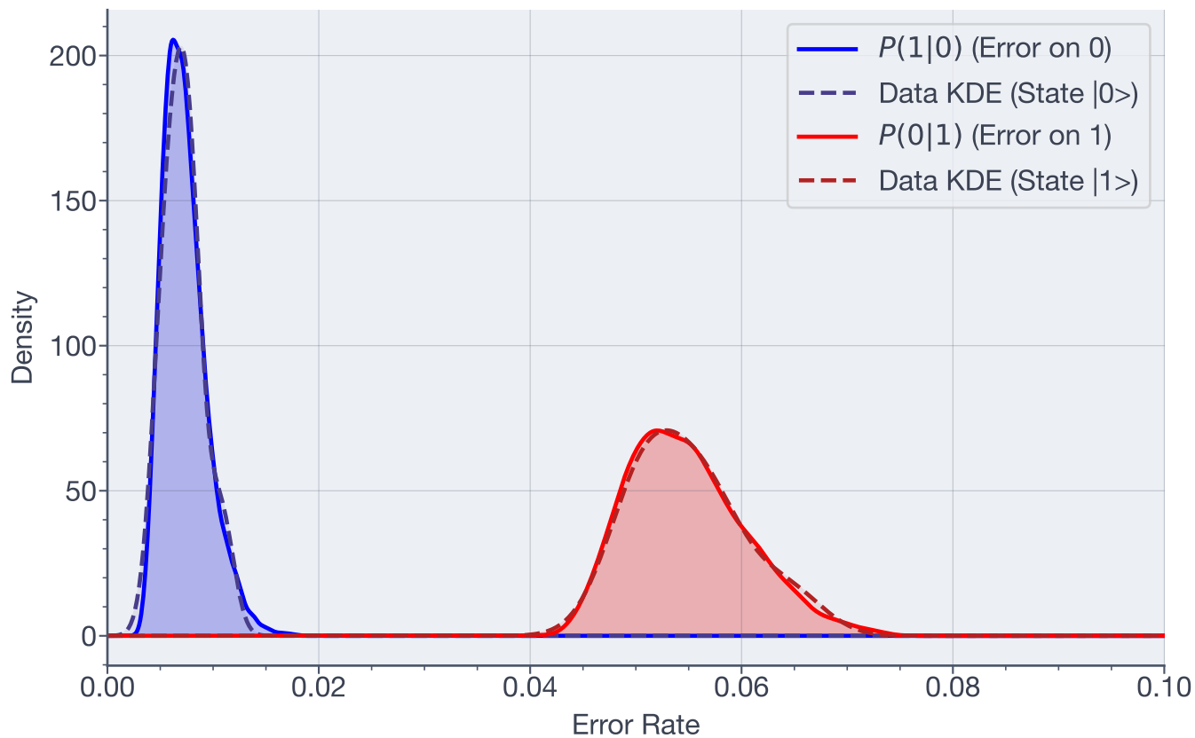
Posterior Error Distributions - Qubit 12
