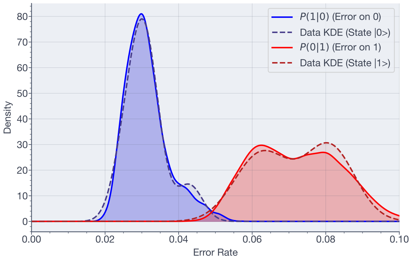
Posterior Error Distributions - Qubit 31
