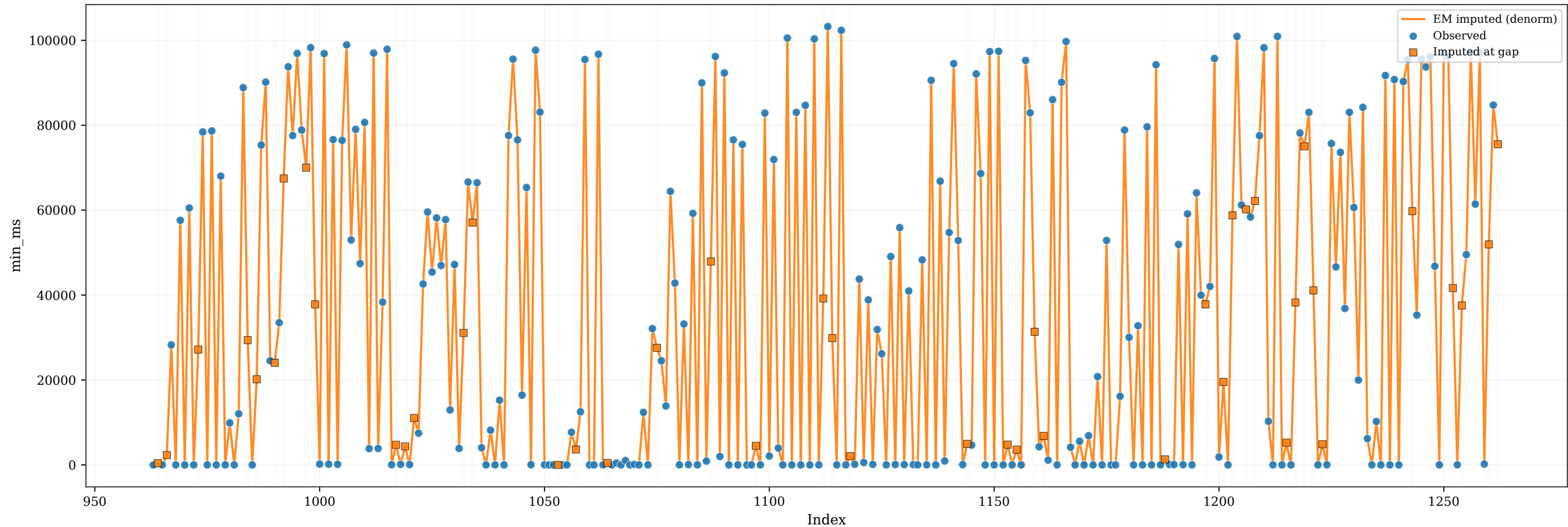
min_ms — Overlay comparison (idx 963-1263)
