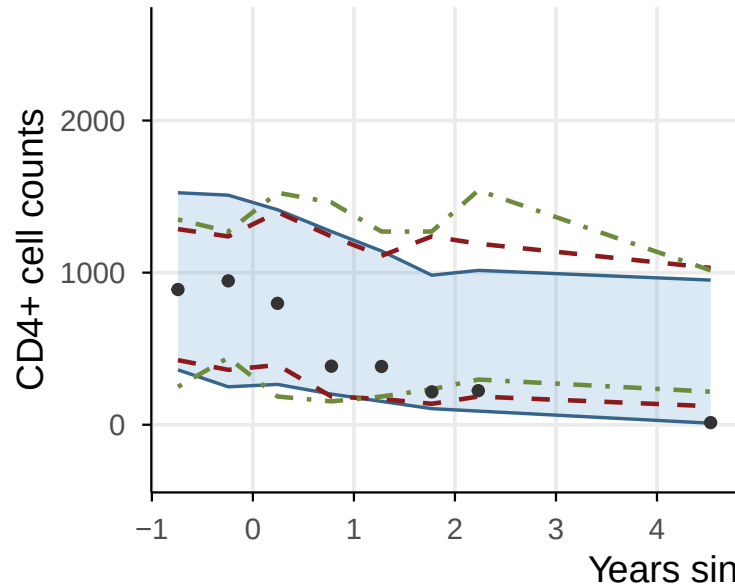
ID = 20344
