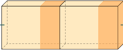
Conv
