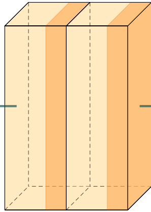
Conv
