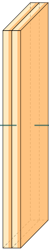
Conv
