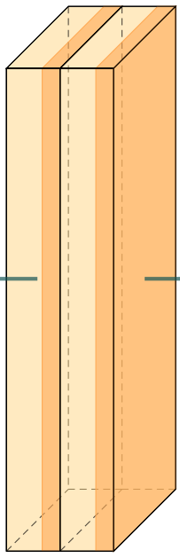
Conv
