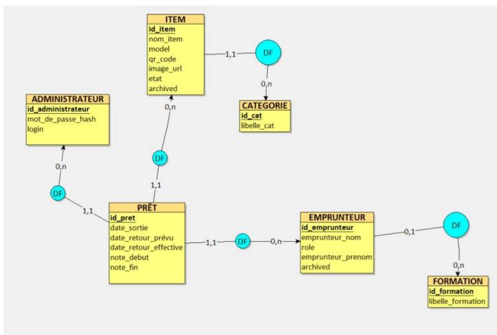
MCD MediaStock – 6 entités : ITEM, CATEGORIE, PRÊT, EMPRUNTEUR, FORMATION, ADMINISTRATEUR
