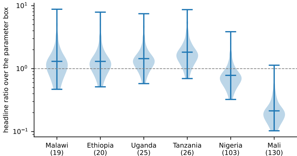
ssp585: 1280 Saltelli points, posterior-median parameters
