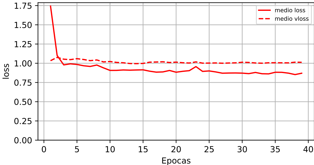
Valor Perdida - Nacional-1
