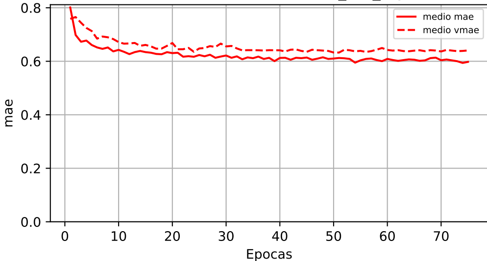
Error absoluto medio - SIMO_asc_ing-1
