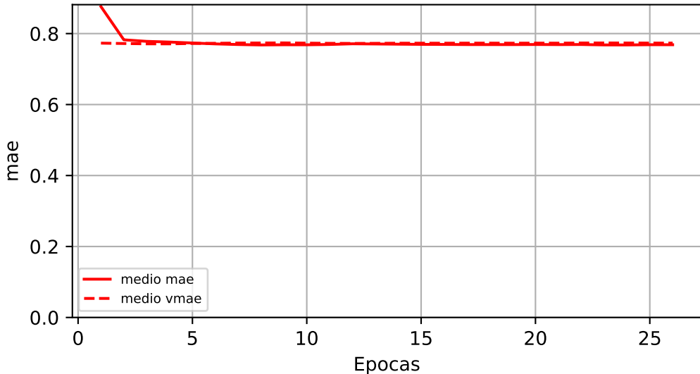
Error absoluto medio - Asistencial-1
