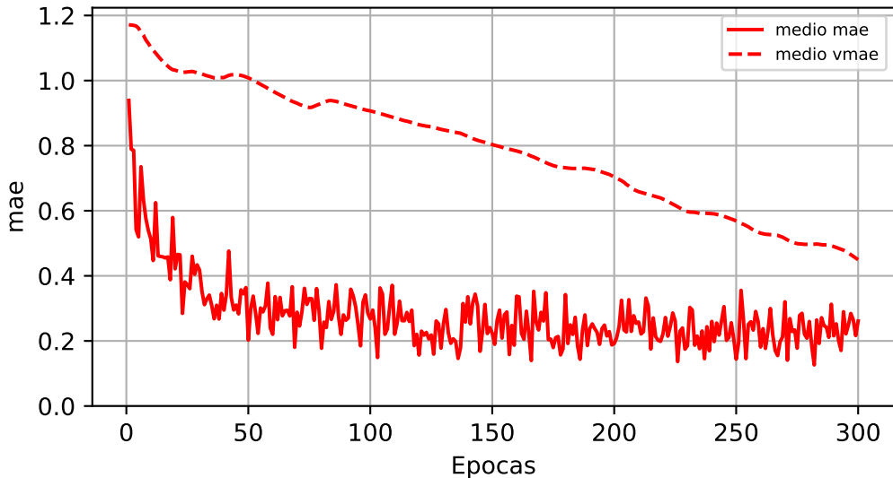
Error absoluto medio - Bomberos-0
