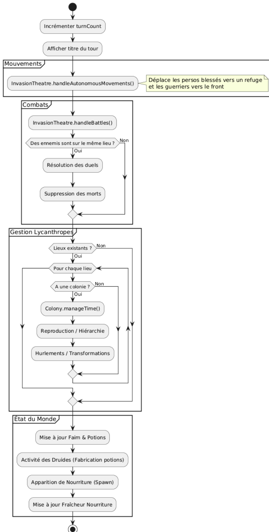
Diagramme de Flux : Déroulement d'un Tour (runNextTurn)
