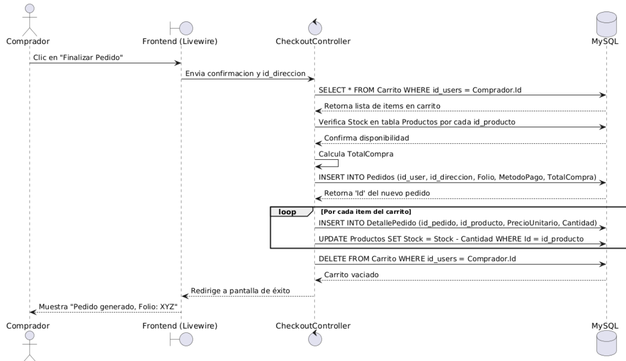
Diagrama 2: Comprador - Realizar pago y finalizar pedido
