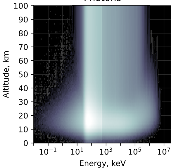
Photons
