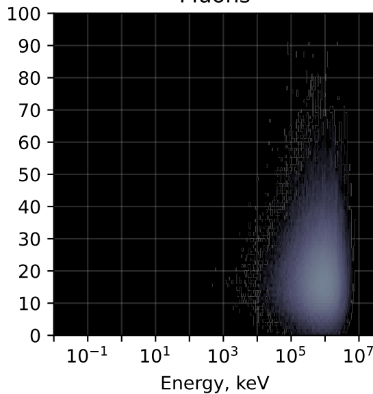
Muons
