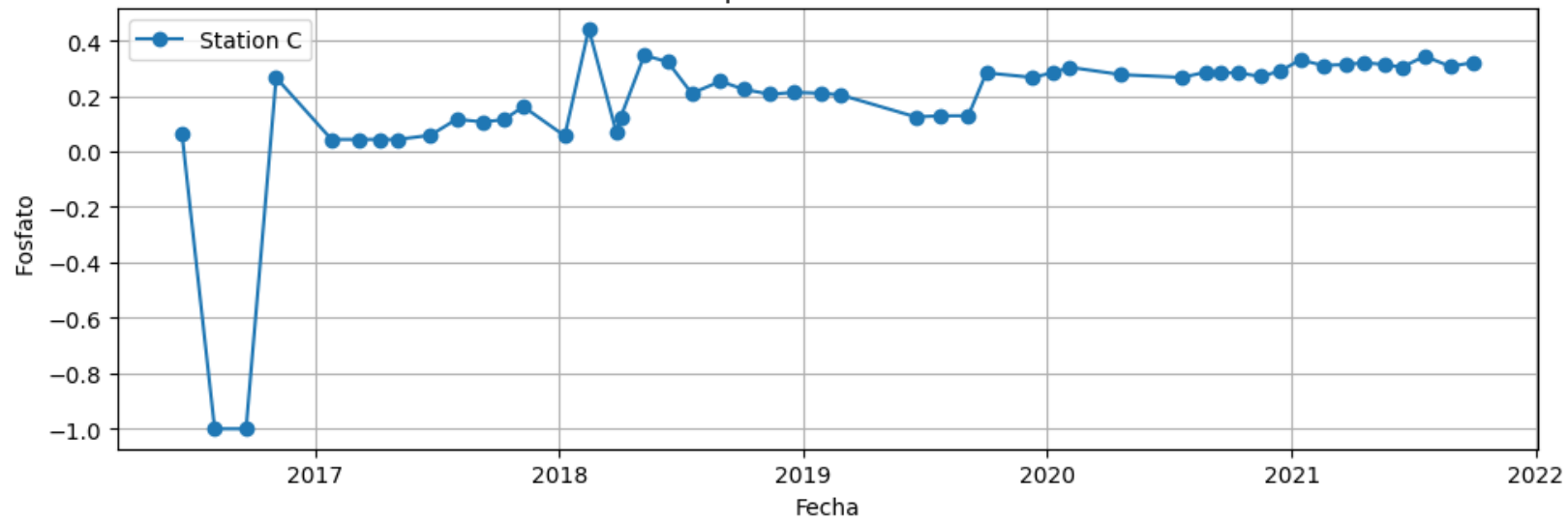
Serie temporal FOSFATO- Station C
