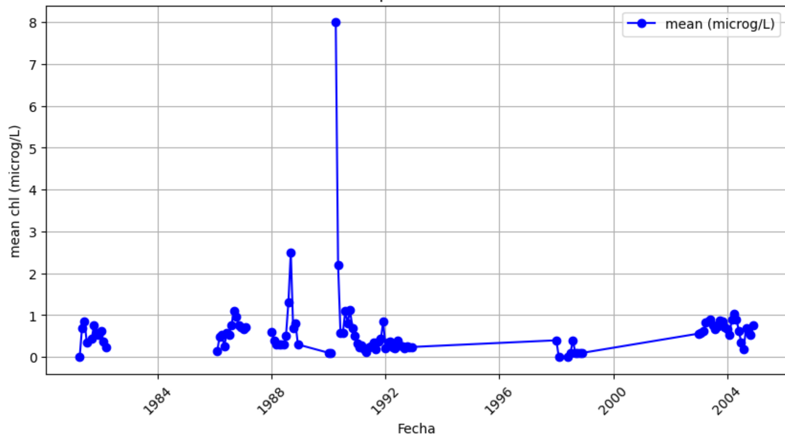
Serie Temporal de la clorofila
