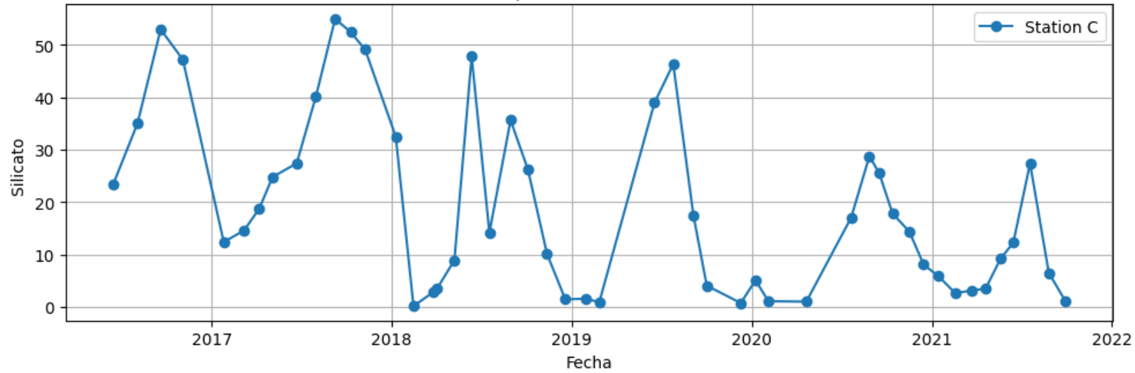
Serie temporal SILICATO- Station C
