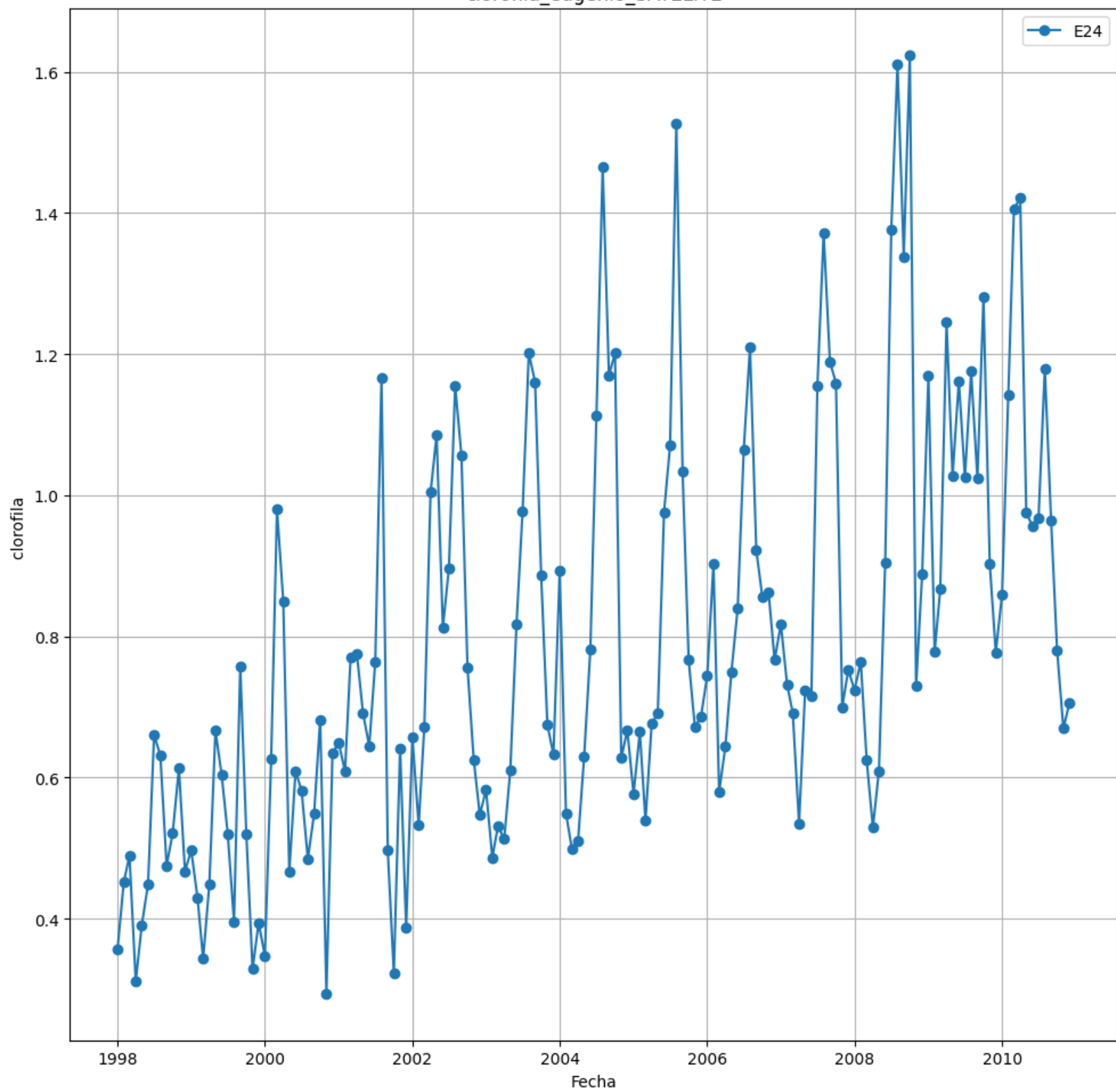
clorofila_eugenio_SATELITE
