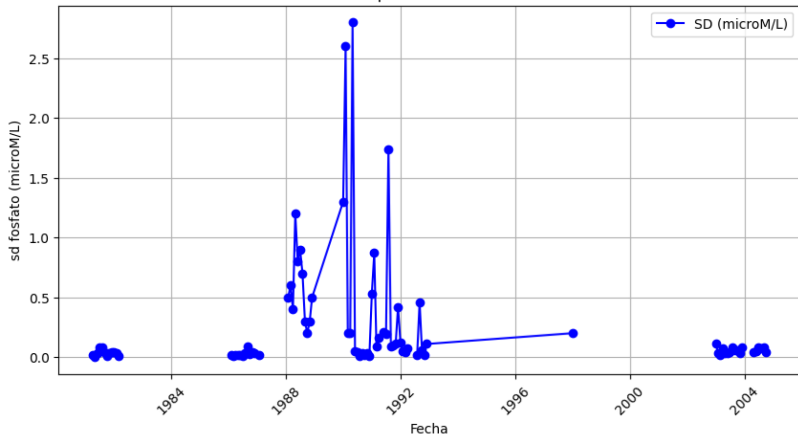
Serie Temporal del sd del fosfato
