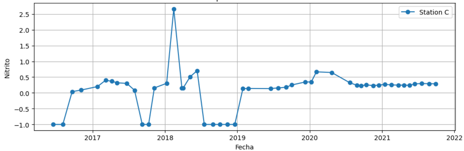
Serie temporal NITRITO- Station C
