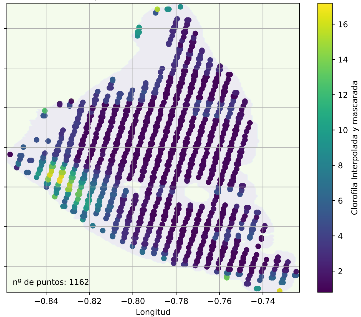
Datos interpolados fecha 2023-08-28 00:00:00
