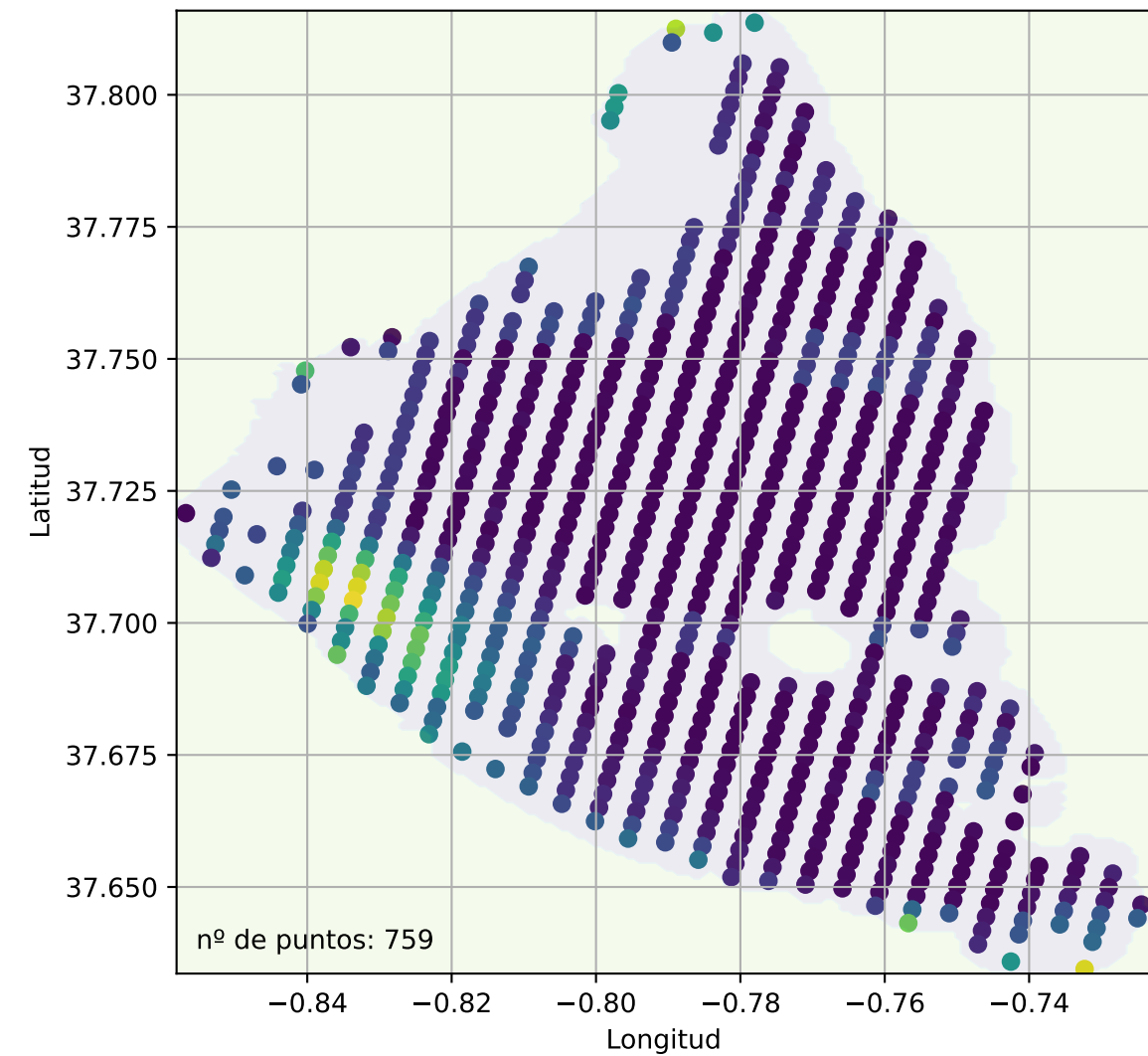
Datos reales fecha 2023-08-28 00:00:00
