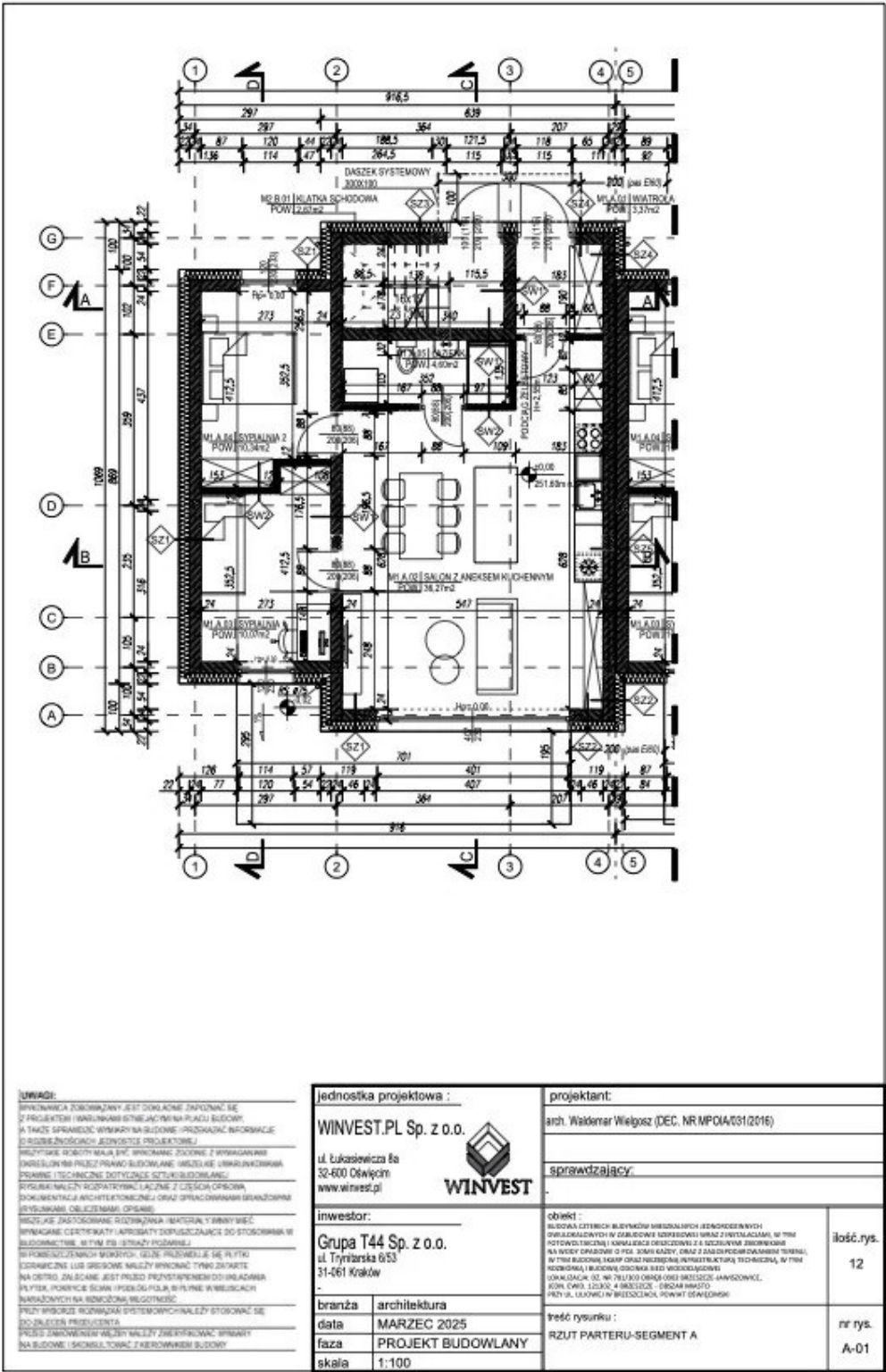
Rysunek z projektu budowlanego, skala 1:100. Układ identyczny dla segmentów A, B i C, segment D stanowi odbicie lustrzane.
