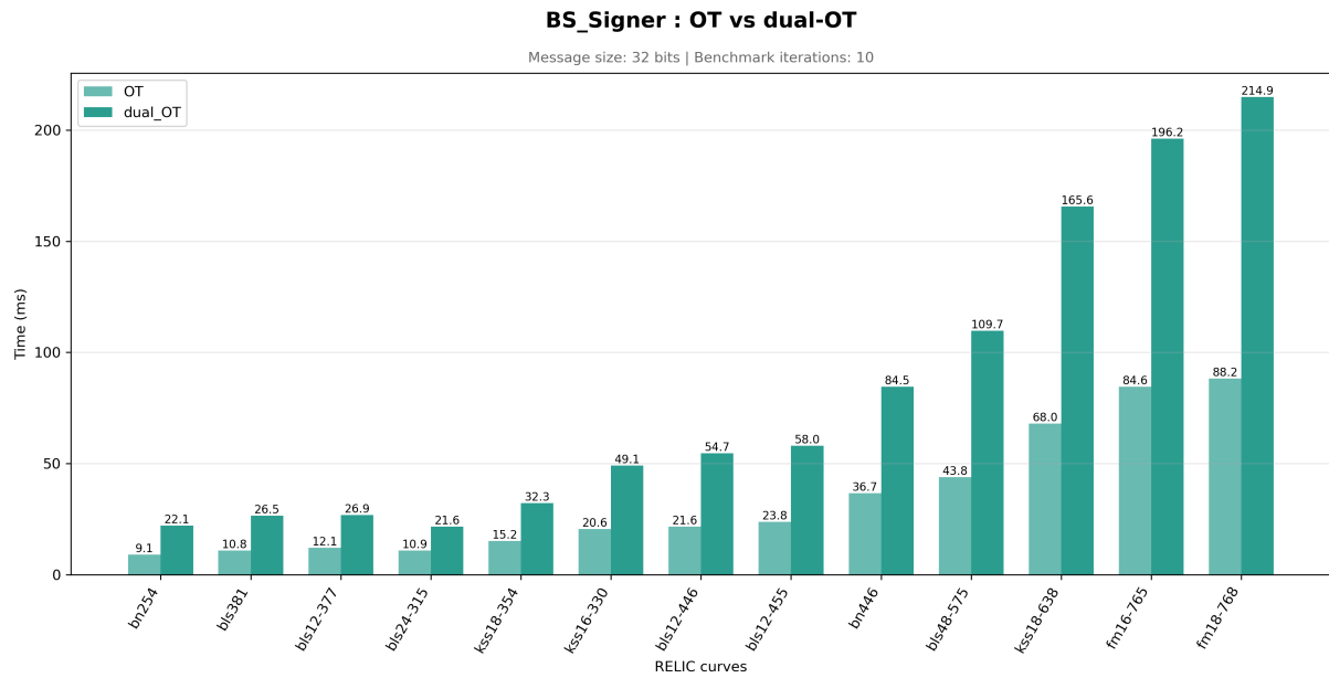
FIGURE 8 – Temps d'exécution de l'étape du signataire pour les protocoles OT et dual-OT.
