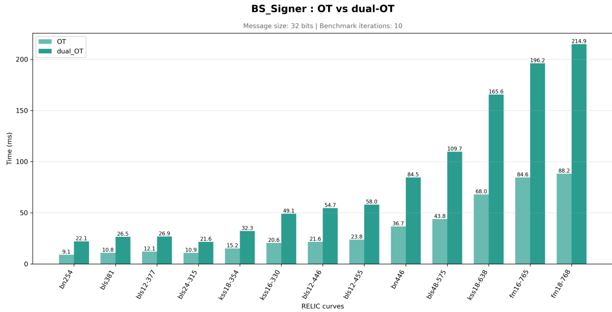
FIGURE 6 – Temps d'exécution de l'étape du signataire pour les protocoles OT et dual-OT.
