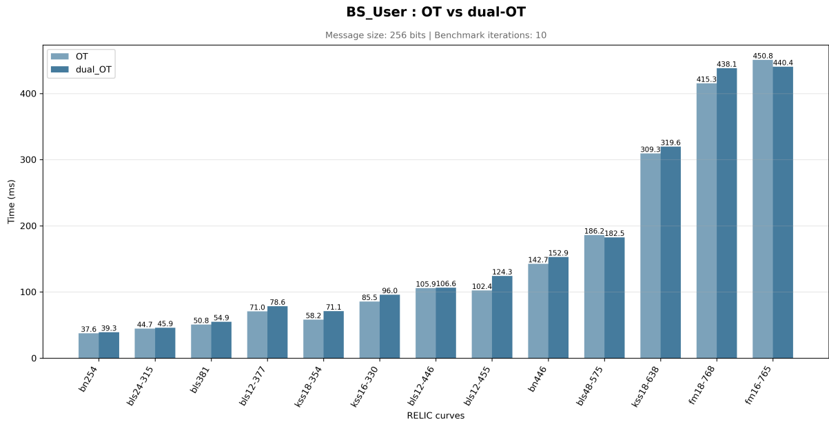
FIGURE 5 – Temps d'exécution de l'étape utilisateur pour les protocoles OT et dual-OT.
