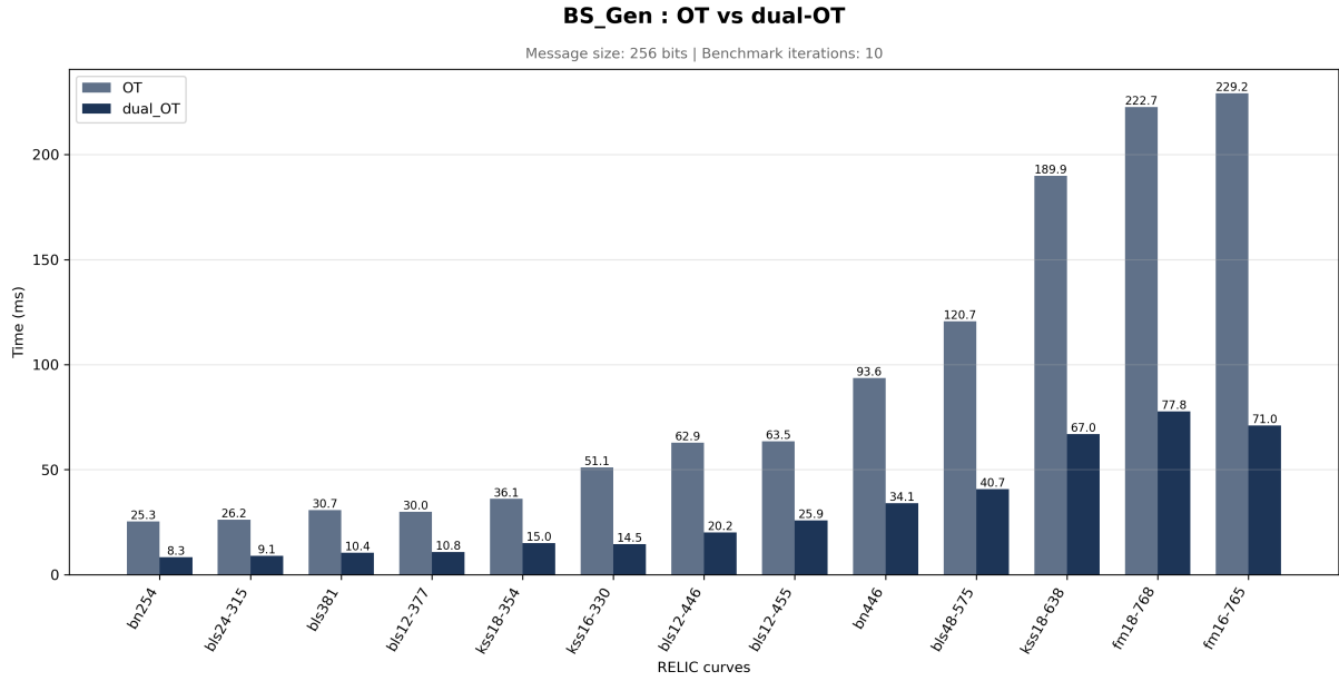
FIGURE 4 – Temps d'exécution de la génération des clés pour les protocoles OT et dual-OT.
