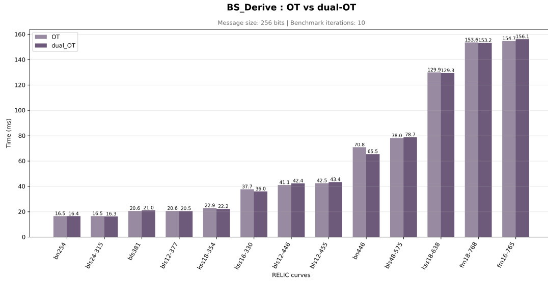
FIGURE 10 – Temps d'exécution de la dérivation de la signature pour les protocoles OT et dual-OT.
