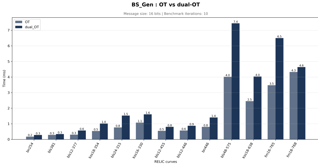
FIGURE 7 – Temps d'exécution de la génération des clés pour les protocoles OT et dual-OT.
