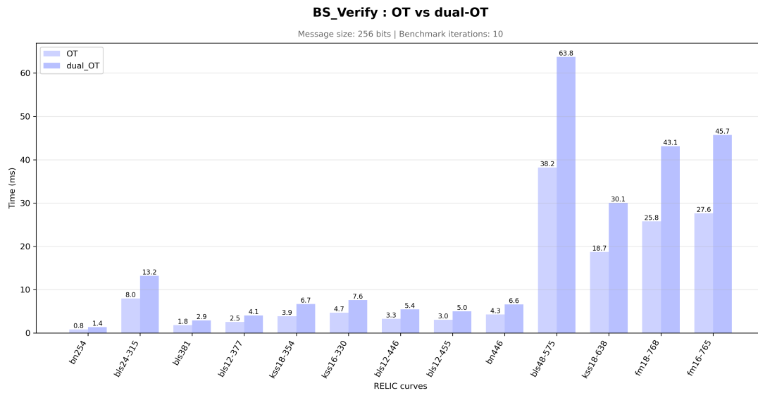
FIGURE 11 – Temps d'exécution de la vérification pour les protocoles OT et dual-OT.
