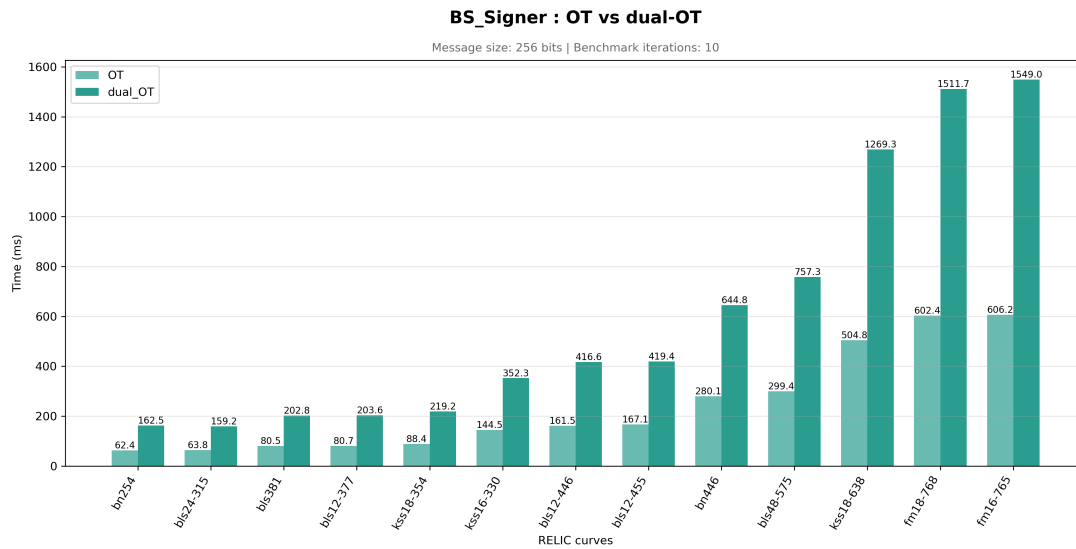
FIGURE 9 – Temps d'exécution de l'étape du signataire pour les protocoles OT et dual-OT.
