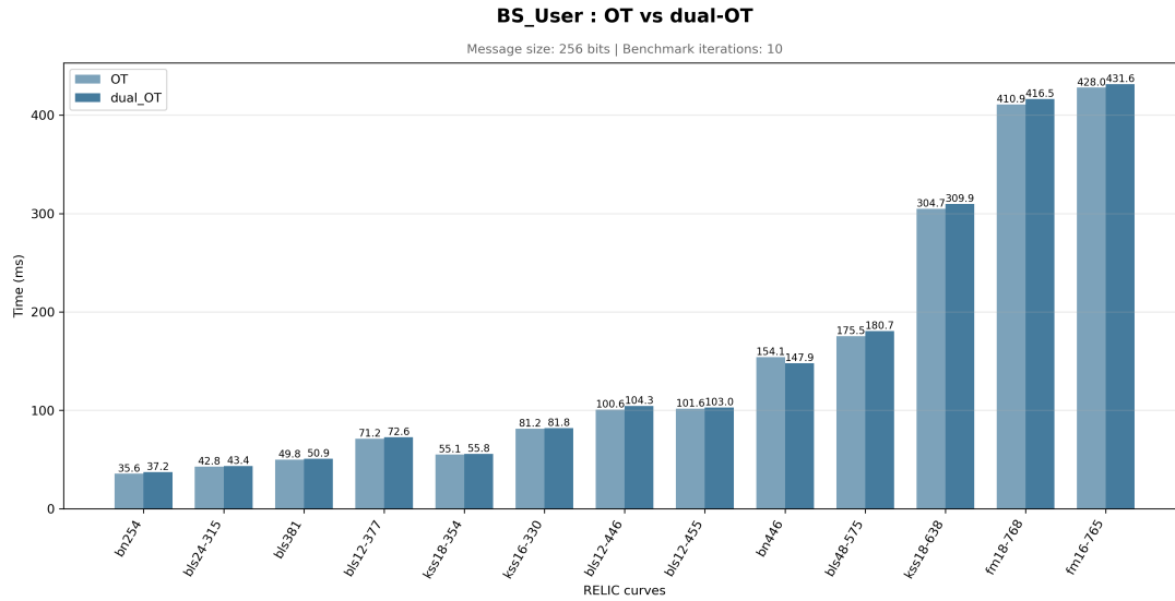
FIGURE 8 – Temps d'exécution de l'étape utilisateur pour les protocoles OT et dual-OT.
