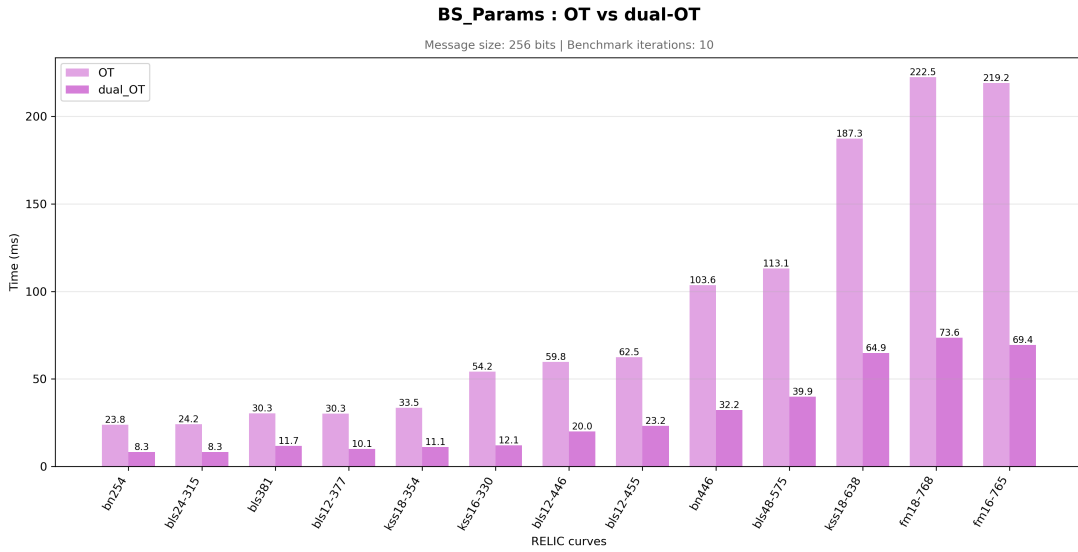
FIGURE 6 – Temps d'exécution de la générations des paramètres publics pour les protocoles OT et dual-OT.
