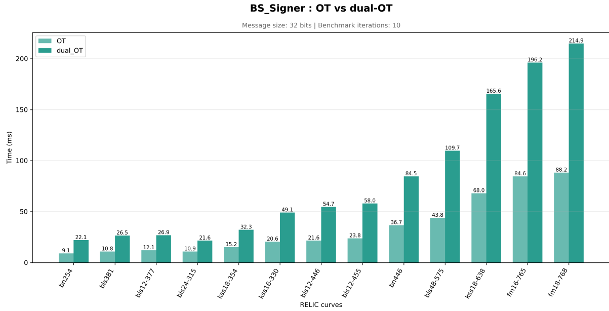
FIGURE 7 – Temps d'exécution de l'étape du signataire pour les protocoles OT et dual-OT.
