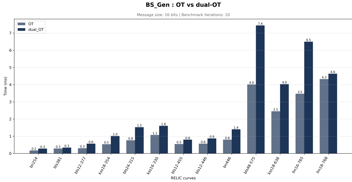
FIGURE 5 – Temps d'exécution de la génération des clés pour les protocoles OT et dual-OT.
