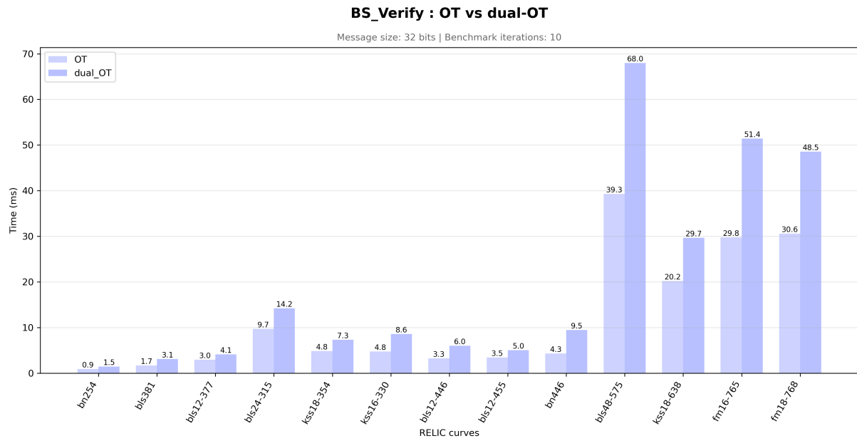
FIGURE 9 – Temps d'exécution de la vérification pour les protocoles OT et dual-OT.
