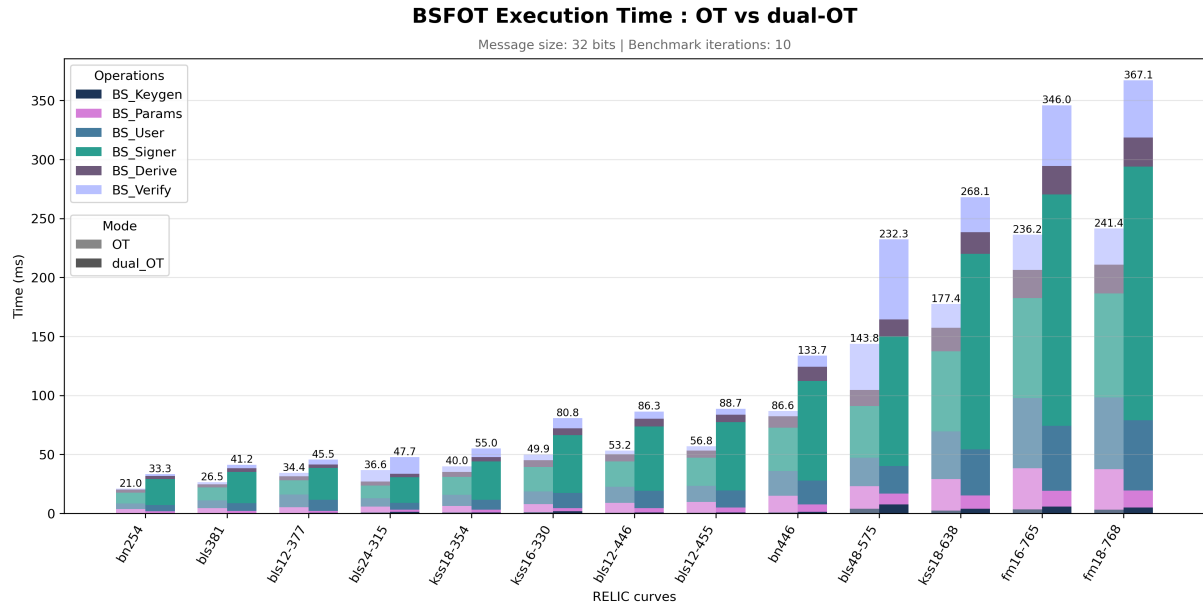
FIGURE 2 – Benchmark global de comparaison entre le protocole OT et le protocole dual-OT pour différentes courbes elliptiques.
