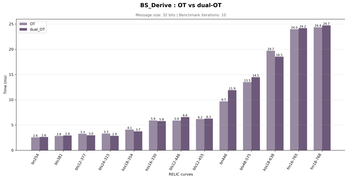
FIGURE 8 – Temps d'exécution de la dérivation de la signature pour les protocoles OT et dual-OT.
