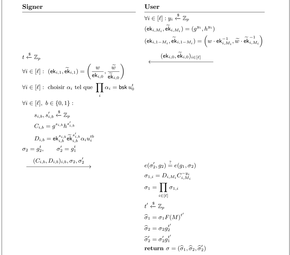
FIGURE 1 – Schéma de signature aveugle basé sur le dual-OT
