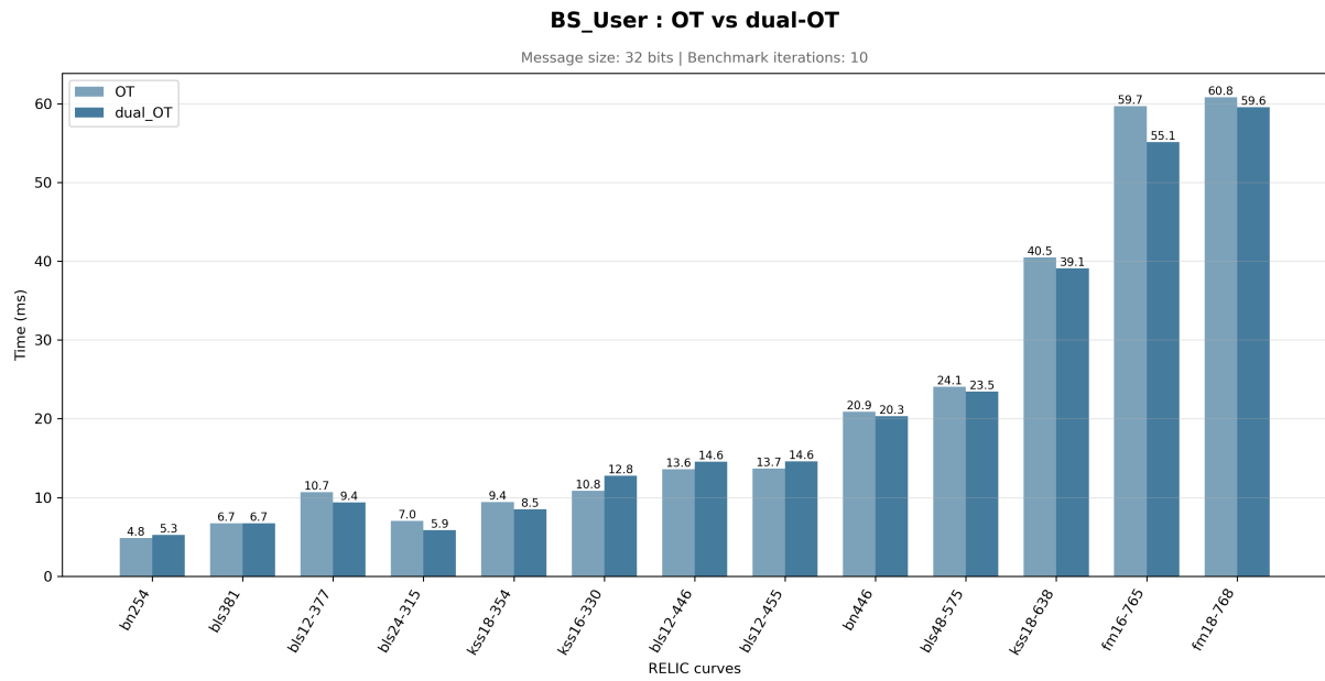
FIGURE 6 – Temps d'exécution de l'étape utilisateur pour les protocoles OT et dual-OT.
