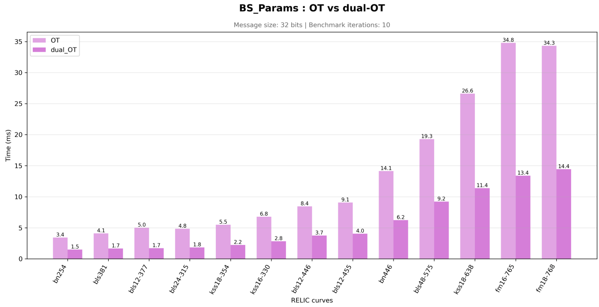
FIGURE 4 – Temps d'exécution de la générations des paramètres publics pour les protocoles OT et dual-OT.
