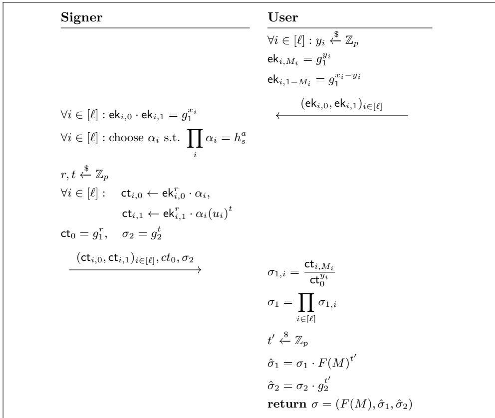
FIGURE 3 – Schéma de signature aveugle basé sur le OT classique
