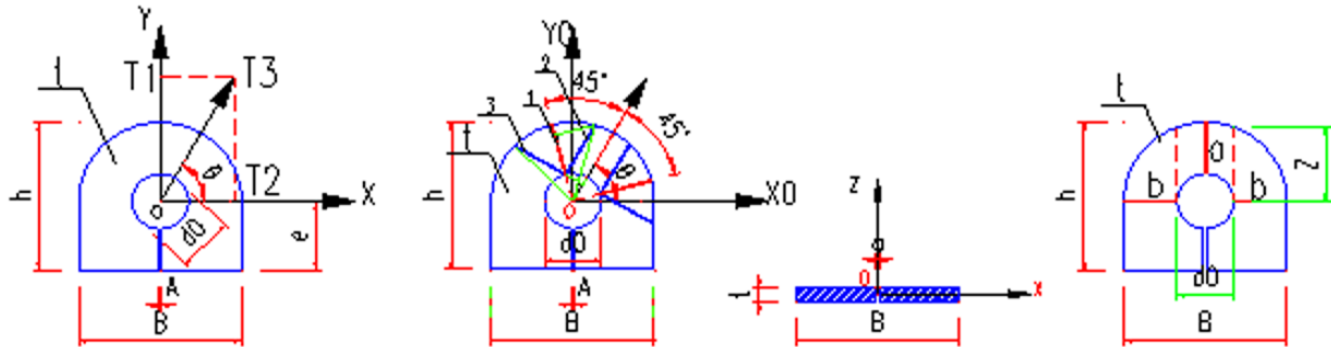
图 1 吊耳尺寸、受力及焊缝计算简图
