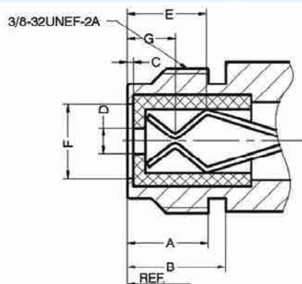
Розетка
