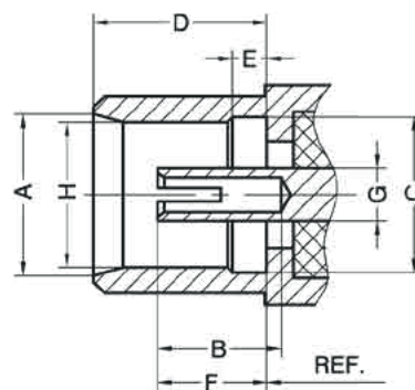
Розетка
