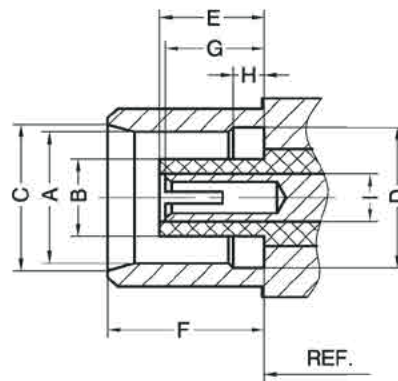
Розетка
