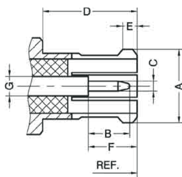
Вилка
