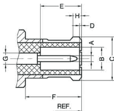
Вилка
