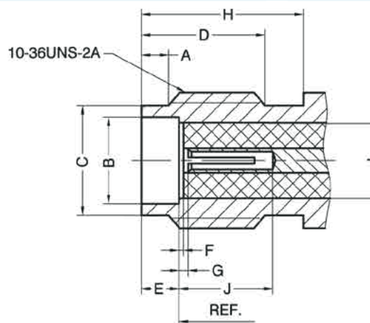
Розетка
