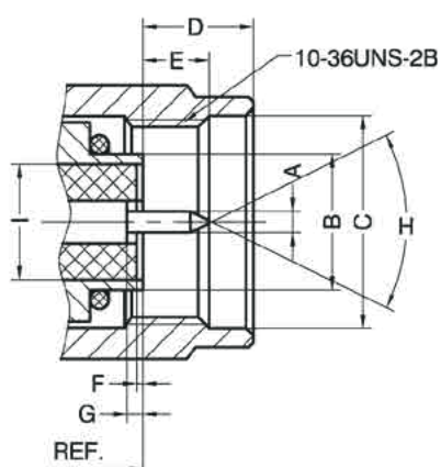
Вилка
