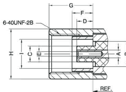
Розетка
