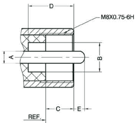
Вилка
