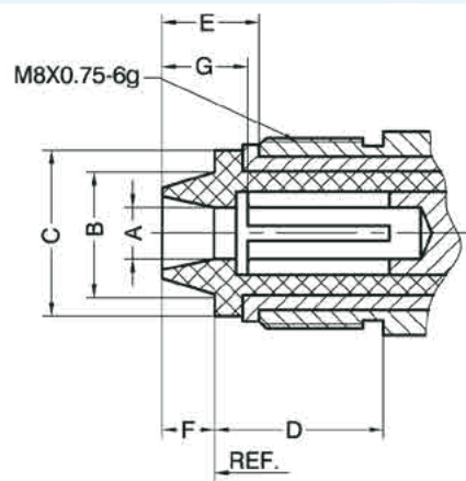
Розетка
