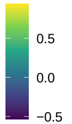
dNBR
