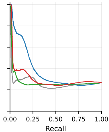
lof
