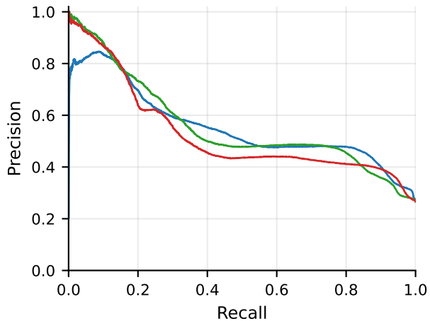
SVM supervisionada
