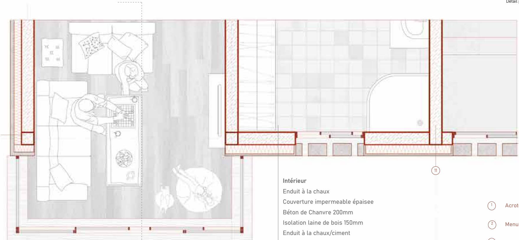
Détail plan 1:20
