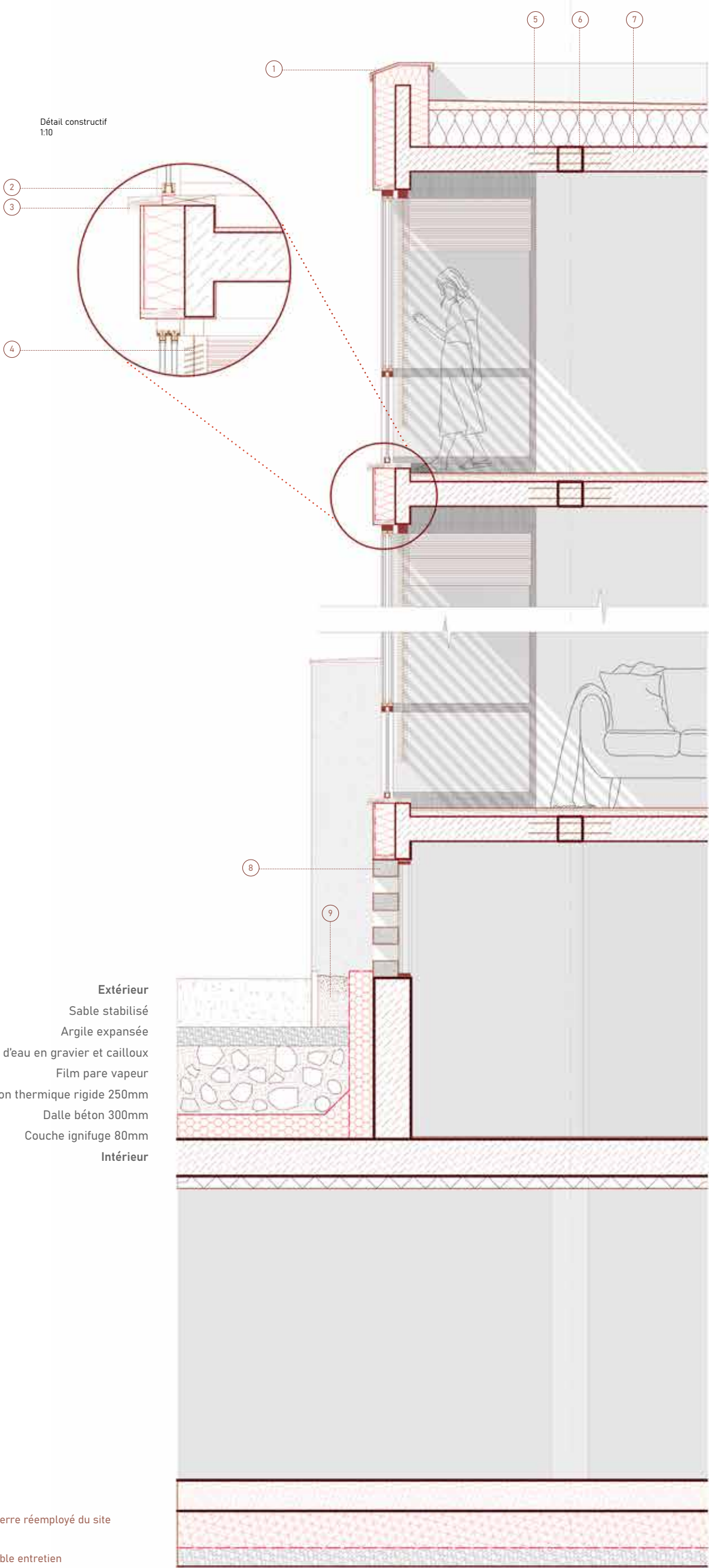
Coup détail - Fenêtre en saillie 1:20
