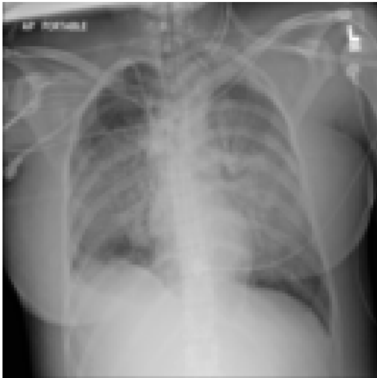
Input
