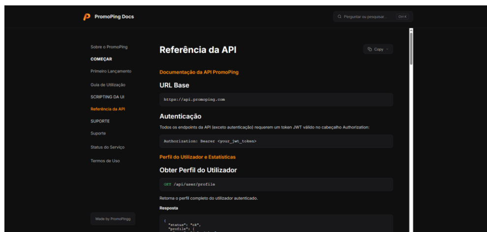
Figura 28- Referencias de API usada no projeto
