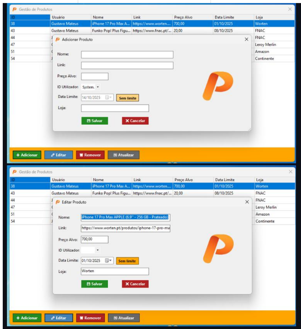
Figura 44- O que há quando clicar nos botões podendo alterar
