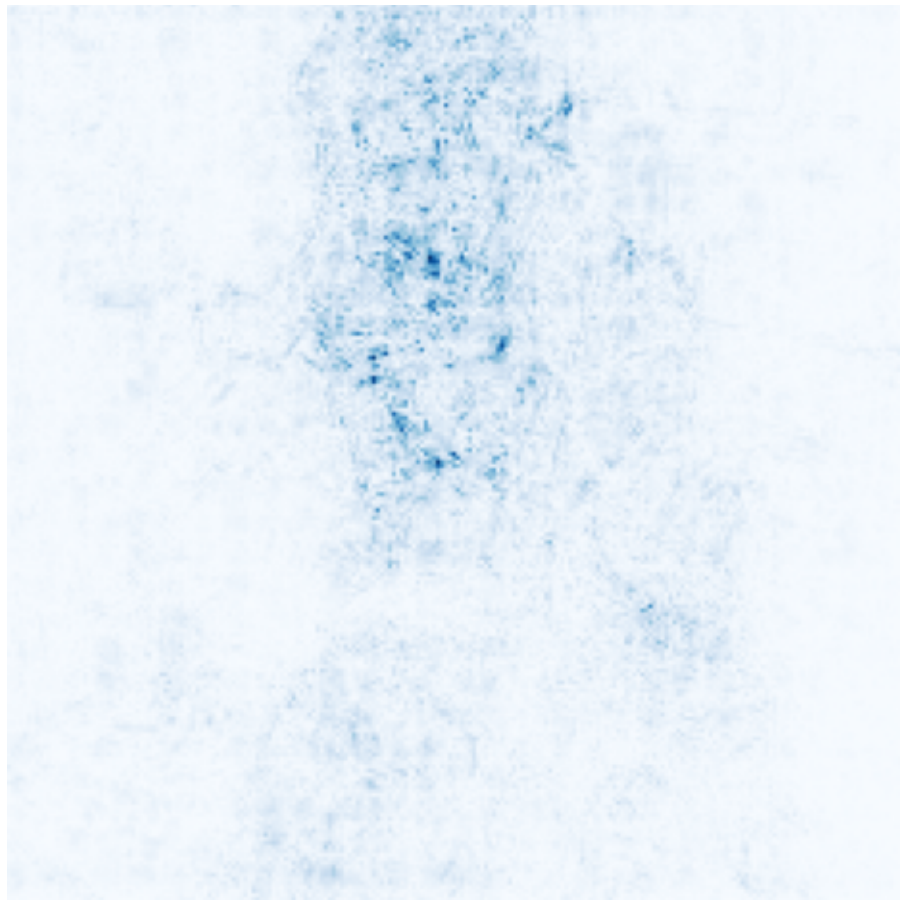
SmoothGrad (n=50)
