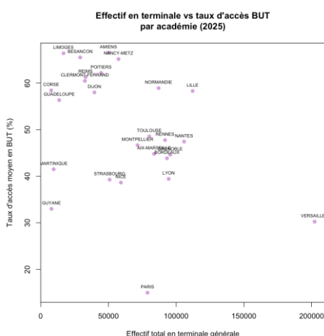
Graphique 5 : Deux variables quantitatives
