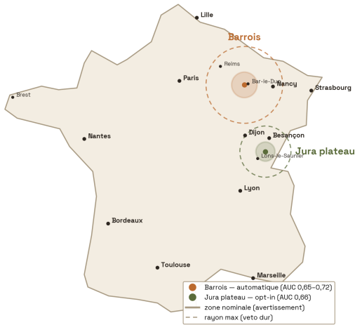
Zones d’application des modèles appris KarstPro
